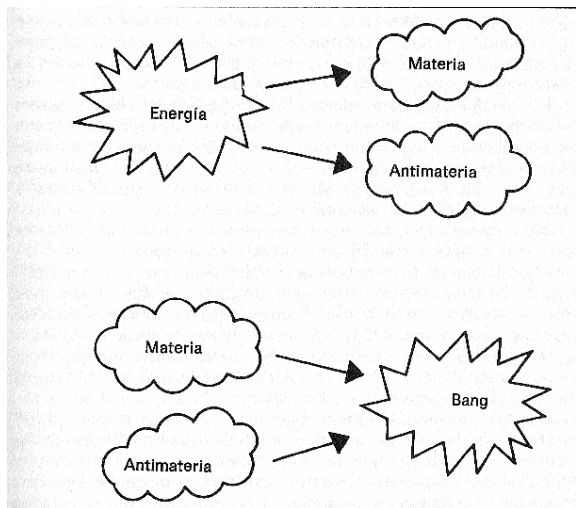
Fig. 4. En el laboratorio se puede crear materia a partir de energía, pero al hacerlo se obtiene también una cantidad igual de antimateria. Cuando la materia y la antimateria entran en contacto, se aniquilan en una explosión, liberando la energía que contienen.
