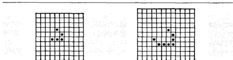
Fig. 26. La simple distribución de cinco puntos conocida como "planeador" tiene la curiosa propiedad de moverse diagonalmente por el tablero, pero permanece intacta. La colección de ocho puntos recibe el nombre de "nave espacial" y también viaja sin sufrir cambio alguno, si bien emite "chispas" a su paso.
