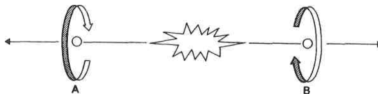
Fig. 11. La desintegración de un átomo o de una partícula subnuclear puede dar lugar a dos partículas (por ejemplo, fotones de luz) que giran en sentido contrario y viajan
