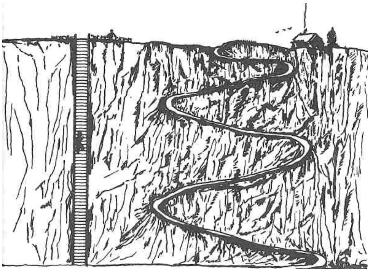
Fig. 24. La ascensión a un acantilado ilustra el concepto abstracto de "simetría de gauge. La energía total necesaria para alcanzar la cima del acantilado es la misma tanto si ascendemos por el camino vertical, corto y cansado, como por la carretera zigzagueante, larga y placentera. Esto es un reflejo de una profunda y potente simetría del campo gravitacional. En recientes formulaciones matemáticas de las teorías de campo unificado se han explotado simetrías semejantes, si bien mucho más complejas, de otros campos de fuerza de la naturaleza.
