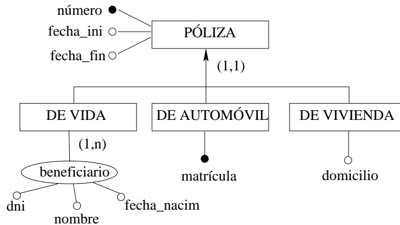
Figura 7.6: Ejemplo de jerarquía de generalización.
