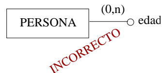
Figura 6.13: No es correcto usar la cardinalidad para expresar el rango de valores.
