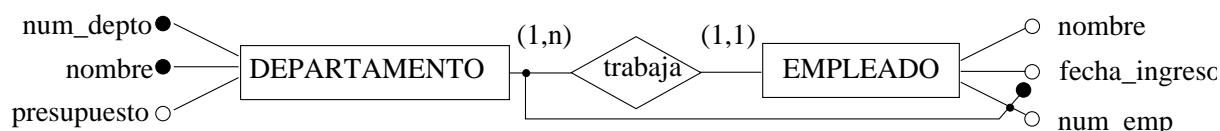
Figura 7.2: Ejemplo de identificador de entidad débil.
