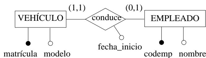
Figura 7.3: Relación de uno a uno.
