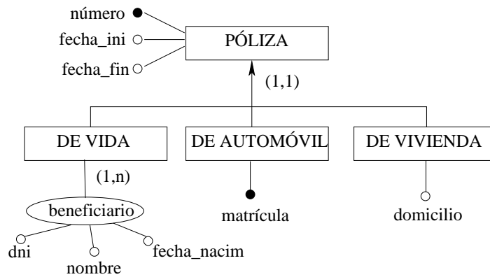
Figura 6.8: Ejemplo de jerarquía de generalización.
