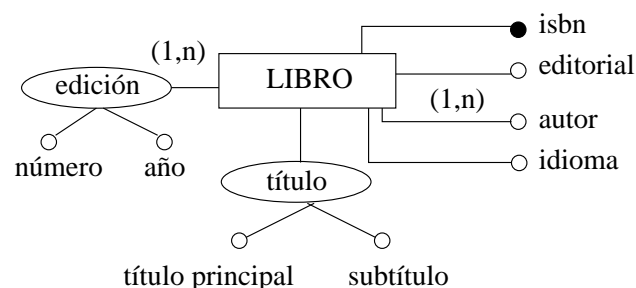
Figura 7.1: Entidad con atributos.
