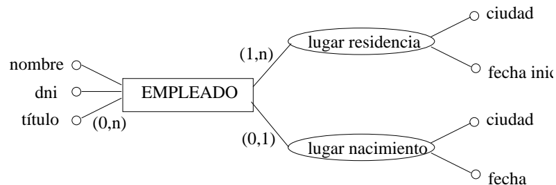
Figura 6.5: Ejemplo de atributos compuestos.
