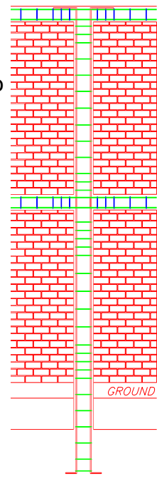
Detalle de la columna de confinamiento en toda su longitud
