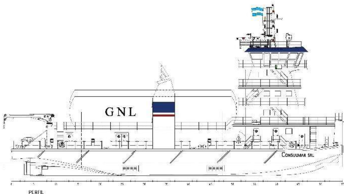
23 - Remolcador de Empuje de GNL, por Consulmar SRL
