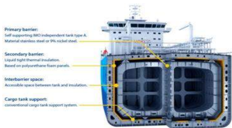
14 - Tanque tipo "A" (LNT)
