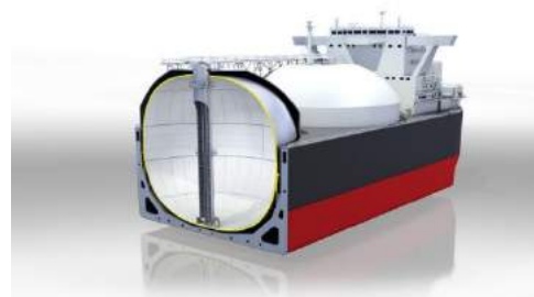
15 - Tanque tipo "B" (KHI).
