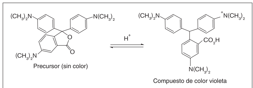
Figura 6. Espirolactonas, que aportan propiedades termocrómicas a los textiles 4 .
