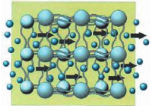
Figura 9. Membrana del material Diaplex por debajo de la temperatura de activación (izquierda) y por encima de ésta (derecha) [26] .
