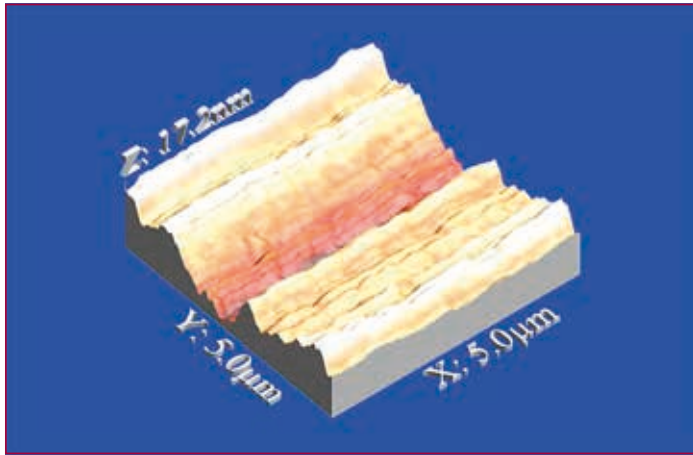
► Figura 5. Rugosidad de superficie de Ti medido por microscopia de fuerza atómica.
