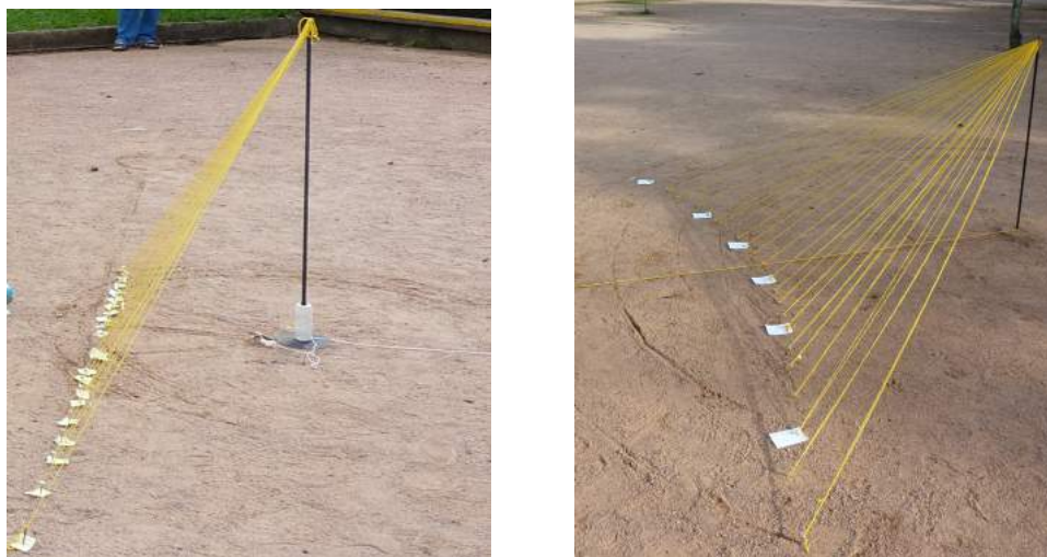
Figura 7.1: Observações com um gnômon em Porto Alegre no equinócio de outono (esquerda) e no solstício do inverno (direita). As linhas amarelas ligam a ponta do gnômon à ponta da sombra nas várias medidas. A sombra mínima dá a direção norte-sul.
