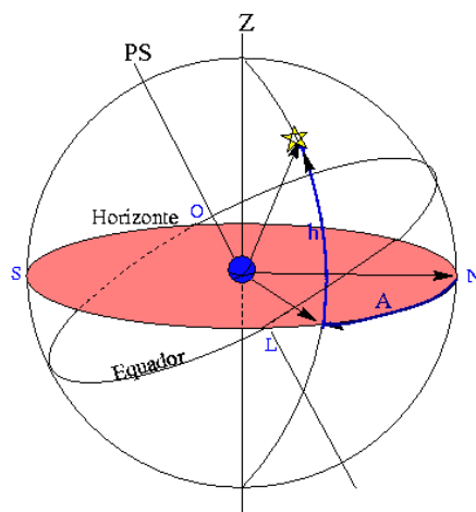
Figura 3.1: Coordenadas do sistema horizontal: altura ( h ) e azimuth ( A ).
