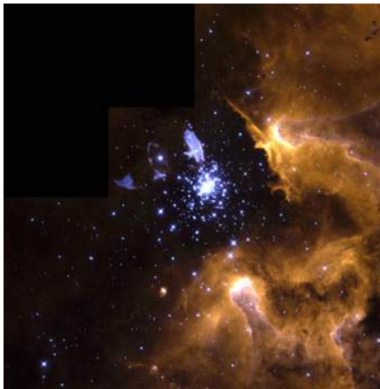
Figura 23.63: Imagem da nebulosa galáctica NGC3603, obtida com o Telescópio Espacial Hubble, mostrando desde estrelas supergigantes e Wolf-Rayet na esquerda, e glóbulos de Bok no canto superior direito.
