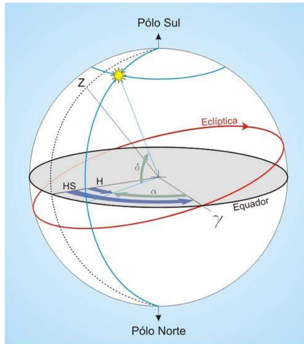
Figura 3.4: O ângulo horário (H) é o ângulo entre o meridiano local (linha pontilhada) e o meridiano do astro (linha azul), contado no sentido do movimento diurno. O ângulo horário do astro somado à sua ascensão reta ( \alpha ), define a hora sideral (HS).
