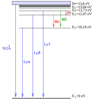
Figura 21.2: Níveis de energia do hidrogênio. Note que o ponto zero da energia é arbitrário e pode ser definido tanto para n=1 quanto para n = \infty .
