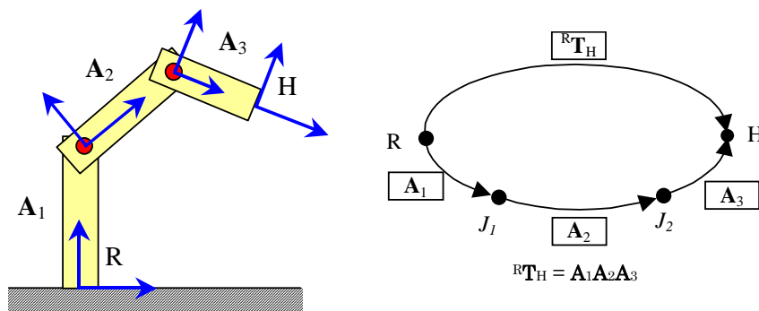
Figura 4.1 - Matriz de transformação de um manipulador série com 3 elos
