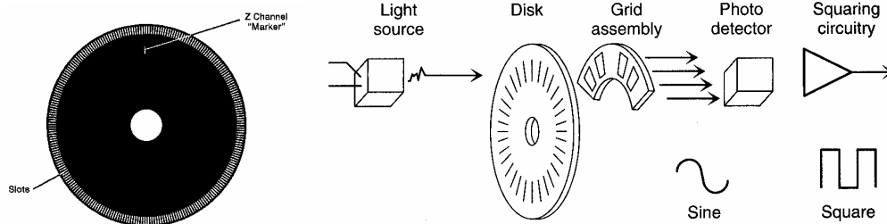
Figura 2.5 - O disco de um codificador óptico relativo e sistema de descodificação relativa (direita)
