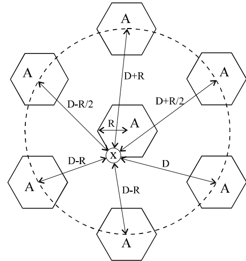
Figura 7 - Ilustração da primeira camada de co-células para cluster com N = 7 . Quando o móvel está localizado no limite de uma célula (ponto X), está sujeito ao pior caso de interferência co-canal no link direto. As distâncias do desenho foram obtidas por simples aproximações
