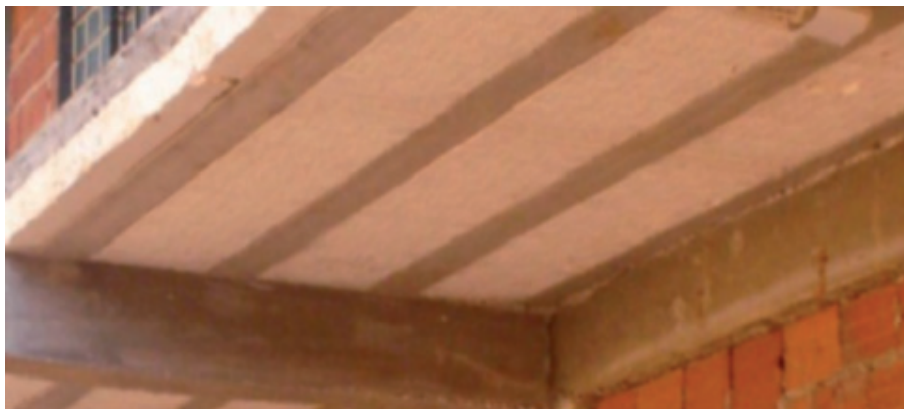
Laje com enchimento de isopor.
