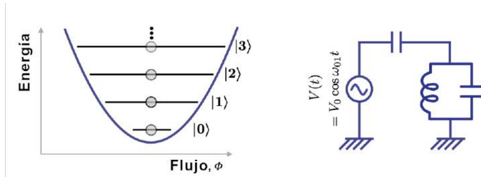
FIGURA 2.2: El el gráfico de la izquierda están representados los diferentes niveles de energía del circuito, en el otro el circuito
