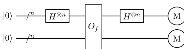
FIGURA 4.4: Circuito de Simon
