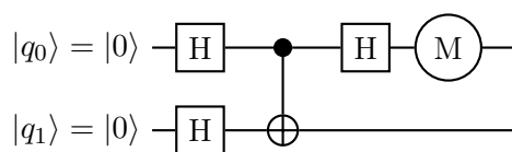
FIGURA 5.7: Circuito de Deutsch y Jozsa
