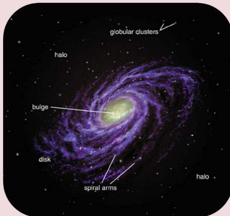
Figura 3: Partes de una galaxia espiral (Créditos: Pearson Education)
