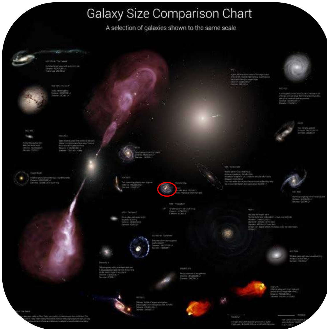
Figura 5: Comparación de tamaños de otras galaxias con la Vía Láctea (rodeada en rojo). (Créditos: rhyisy.net)
