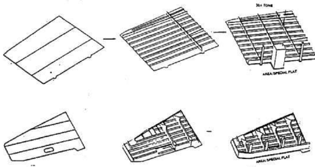
Figura 5 Montagem de painéis
