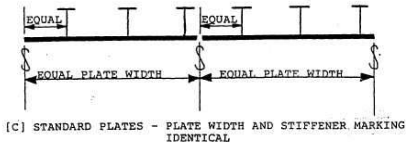
Figura 18 Normalização das chapas
