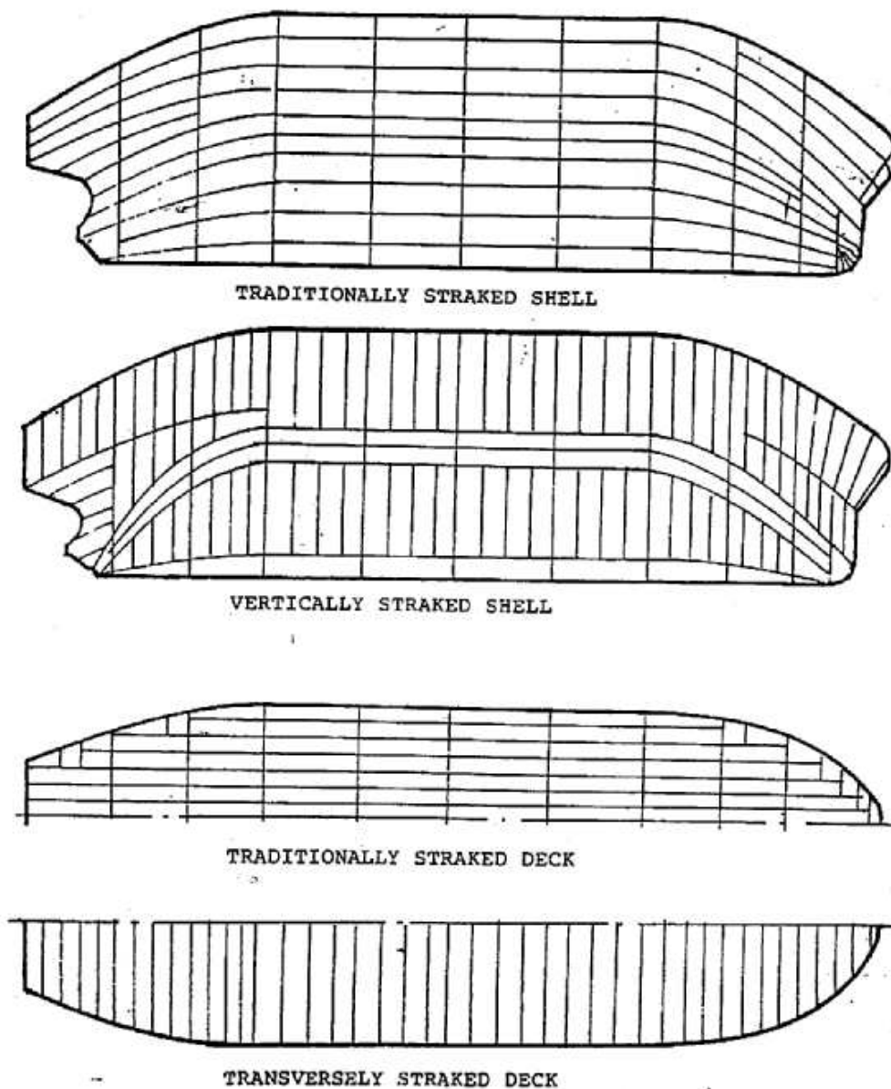
Figura 12 Distribuição das chapas
