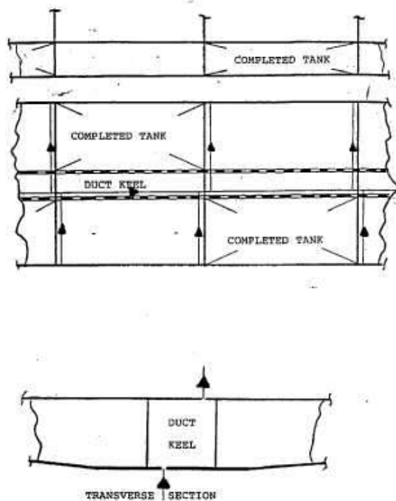
Figura 10 Utilização de coferdames na ligação entre blocos
