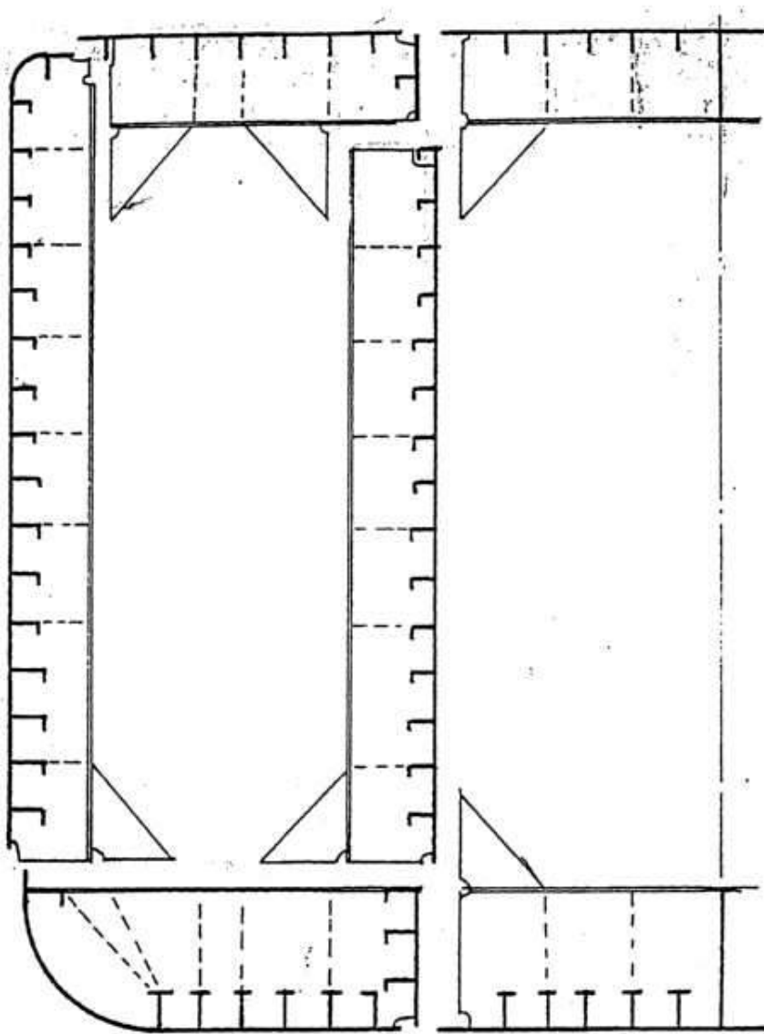
Figura 17 Método de construção em camadas
