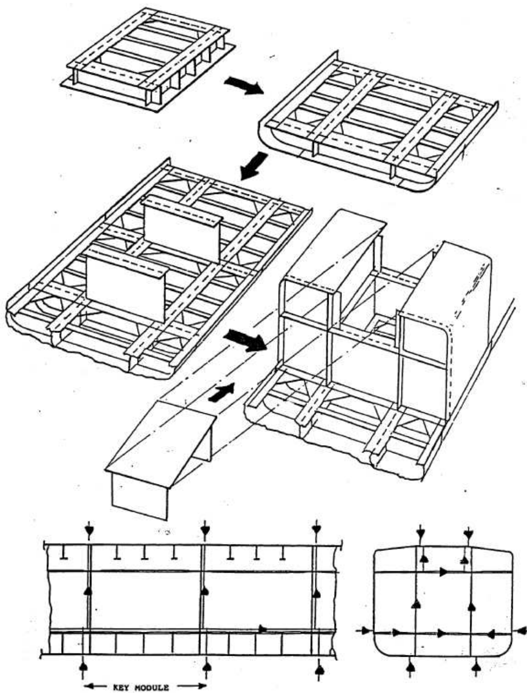
Figura 15 Método de construção em camadas
