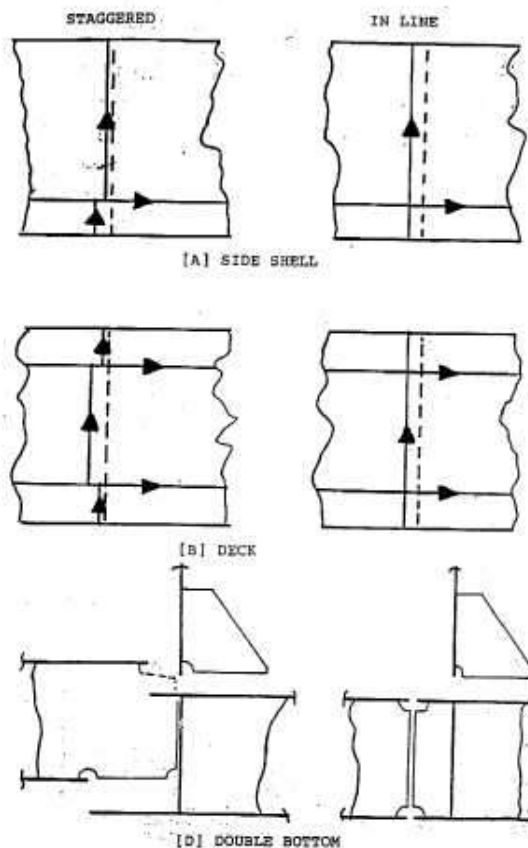
Figura 8 Ligação de blocos
