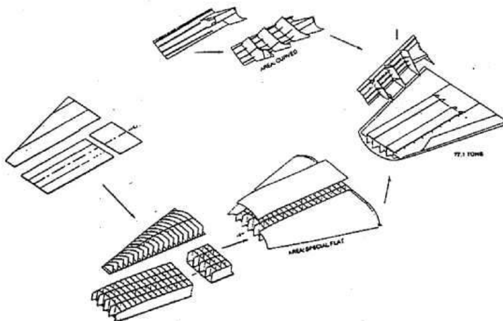
Figura 7 Montagem de Blocos (Roda de Proa)
