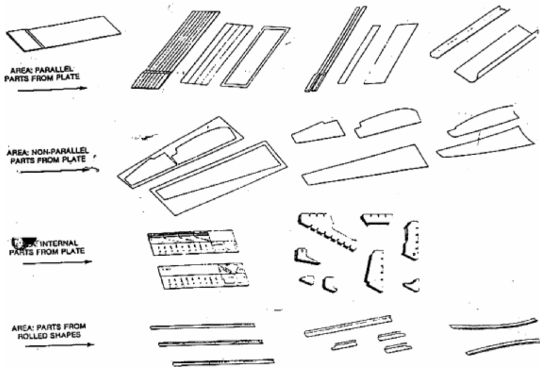
Figura 2 Fabricação de peças
