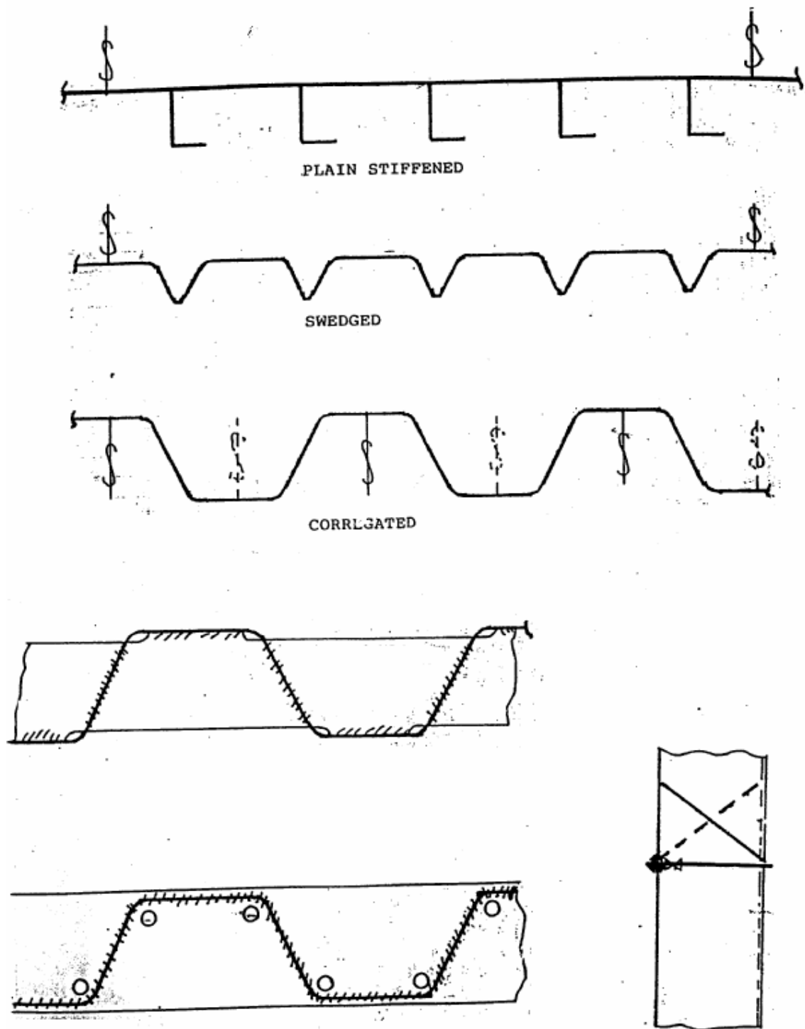
Figura 21 Painéis corrugados e canelados
