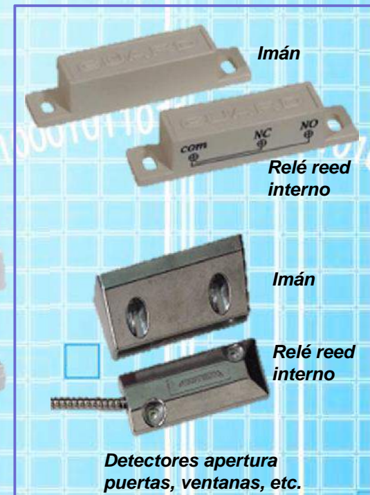
Relé 'reed'
