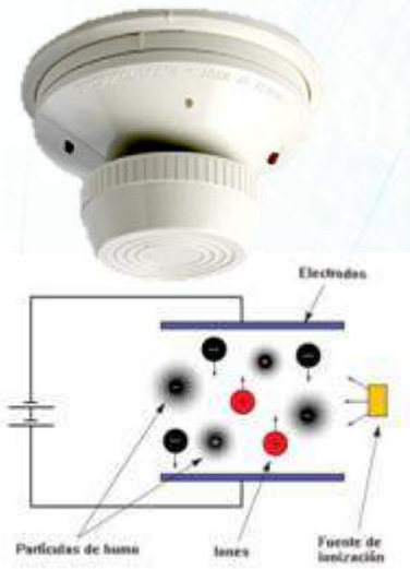
Detector iónico de humo
