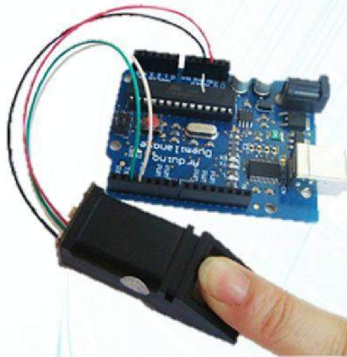
Detector de huella digital
