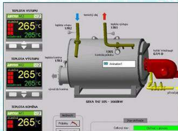
Software de interfaz usuario – Hogar y edificio inteligente (pantalla de calderas)
