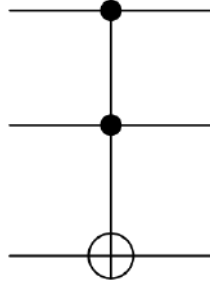
Figura 3.11: Representação circuital da Porta Toffoli Quântica. As linhas superiores representam os q-bits de controle, e a linha de baixo o q-bit-alvo.
