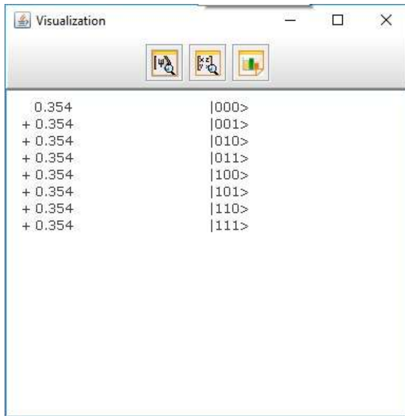
Figura 5.6: Tela do resultado, tipo ket, do Zeno para TFQ.
