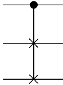
Figura 3.13: Representação circuital da Porta Fredkin Quântica. A linha superior representa o q-bit de controle, e as linhas de baixo os q-bits-alvo.
