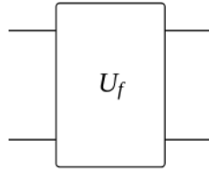
Figura 3.14: Representação circuital de uma Porta Oráculo.
