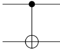
Figura 3.10: Representação circuital da Porta CNOT Quântica. A linha superior representa o q-bit de controle, e a linha de baixo o q-bit-alvo
