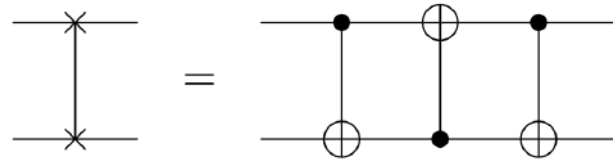
Figura 3.12: Representação circuital da Porta Swap Quântica.
