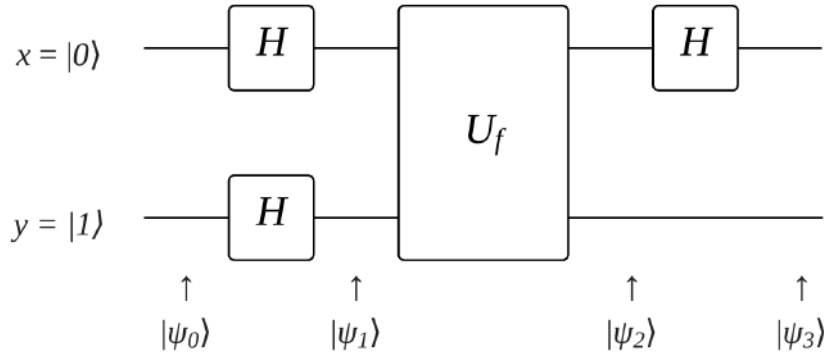
Figura 4.2: Representação de um Circuito de Deutsch.
