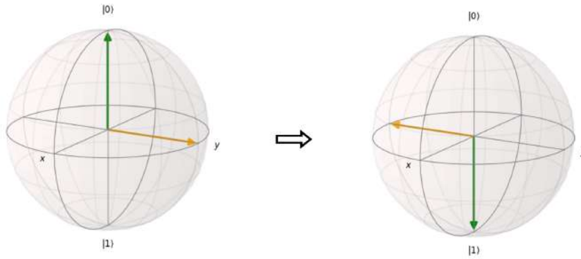
Figura 3.3: O estado do q-bit antes e depois da porta Pauli-X [Gra18].
