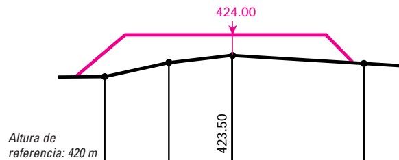
Perfil transversal 175
