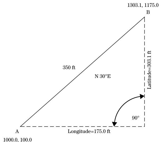
Figure 1-13 Calculating horizontal latitude and longitude coordinates from survey data
