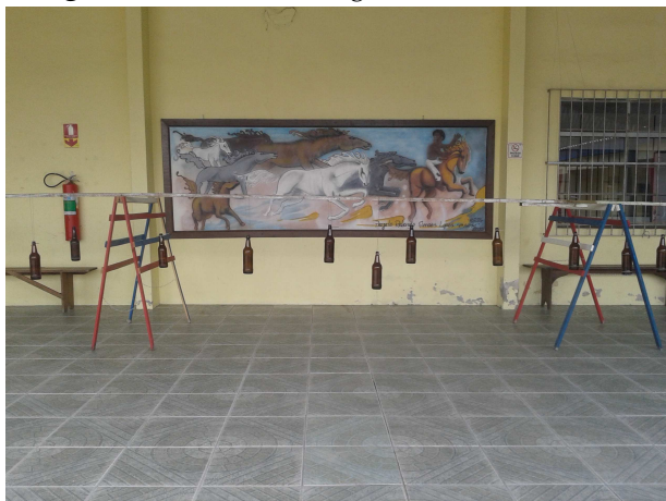
Figura: 1.5. Xilofone de garrafas - visão frontal
