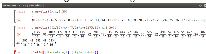
Figura: 2.18. Define gráfico
