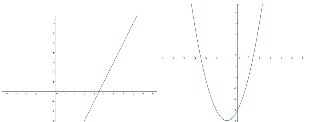
Figura: 5.2. Exemplos de gráficos de função afim e de função quadrática
