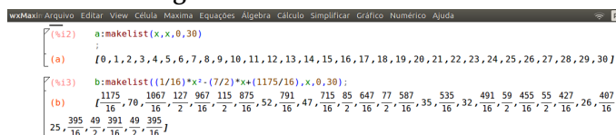
Figura: 2.17. Define listas a e b
