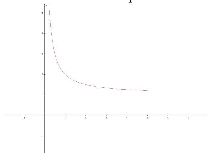
Figura 2.4. Gráfico de g(x) = \frac{x+1}{x} com D(g) = \mathbb{R}_+
