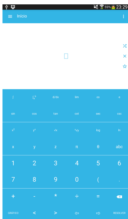
Figura: 4.2. Tela inicial de apresentação.
