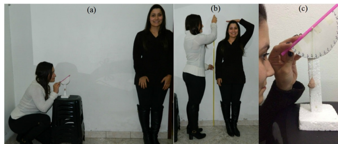
Figura: 3.11. (a) Determinação da altura, com auxílio do teodolito construído. (b) Altura medida com auxílio de trena (c) Ângulo obtido na visada com o teodolito
