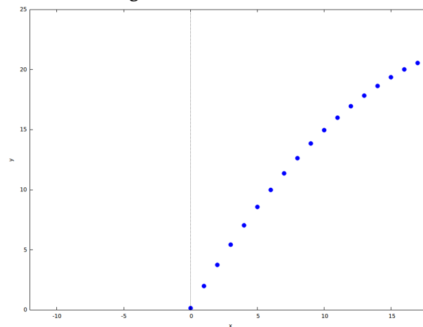
Figura: 2.28. Gráfico solicitado
