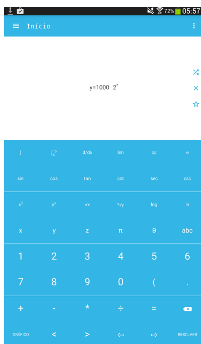
Figura: 4.5. Digitação da expressão y = 1000 \cdot 2^x .
