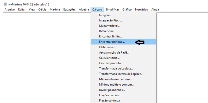
Figura: 2.11. Encontrar ponto de mínimo
