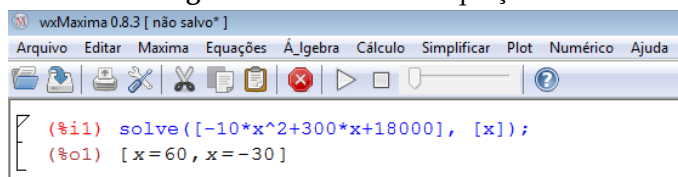
Figura 2.31. Raízes da equação
