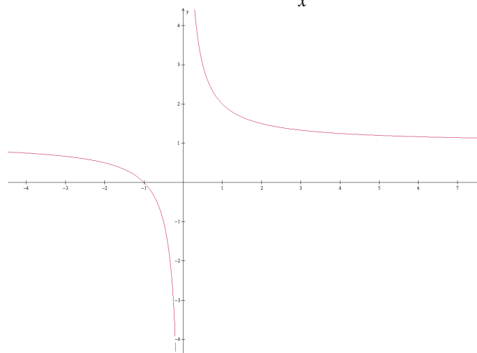
Figura 2.3. Gráfico de f(x) = \frac{x+1}{x} com D(f) = \mathbb{R}^*
