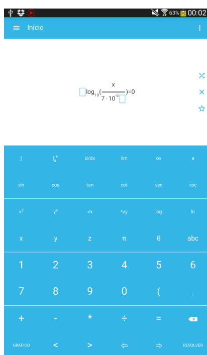
Figura: 4.3. Digitação da equação \log_{10}\left(\frac{x}{7 \cdot 10^{-3}}\right) = 0 .
