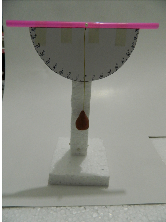
Figura: 3.10. Teodolito finalizado.
