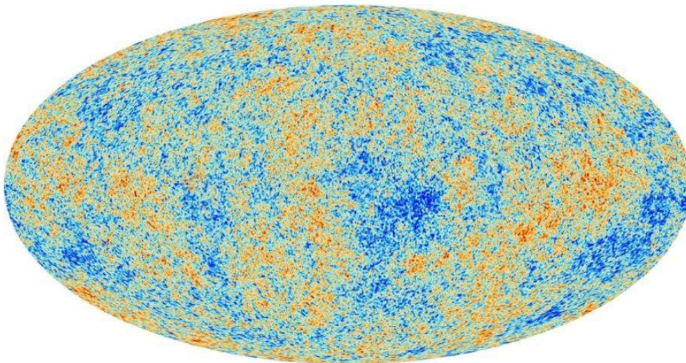
Ilustración 2: Imagen que muestra el fondo de microondas, detallado mapa de todo el cielo del Universo infante, creado con la información de siete años de observaciones del WMAP. La imagen revela fluctuaciones en la temperatura da alrededor de 200 microKelvin (visibles como diferencias de colores) que corresponden a las semillas que llegarían a formar las galaxias. Ha sido sustraída la fuerte señal de nuestra galaxia mediante información de multifrecuencia. Crédito: NASA / WMAP Science Team
