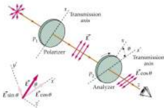
Figura 33.35. Dos láminas polarizadoras con sus ejes de transmisión formando un ángulo \theta . La segunda lámina transmite solamente la componente E \cos \theta . Si la intensidad entre láminas es I_0 , la transmitida finalmente es I_0 \cos^2 \theta .
