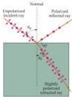
Figura 33.37. Polarización por reflexión. La onda incidente no está polarizada y tiene componentes de E paralela al plano de incidencia (flechas) y perpendicular (puntos). Si el ángulo incidente es el de Brewster, la onda reflejada está totalmente polarizada, con E perpendicular al plano de incidencia (polarización s ).
