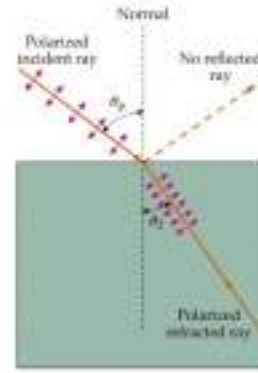
Figura 33.38. Luz polarizada incidente con el ángulo de Brewster: no hay rayo reflejado. La polarización p , paralela al plano de incidencia se representa por flechas. La polarización perpendicular s por puntos.
