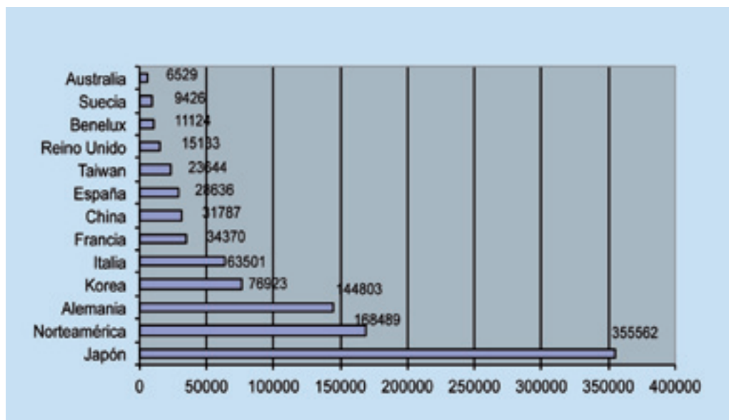
Figura 4.3: Parque mundial de robots en 2008.
