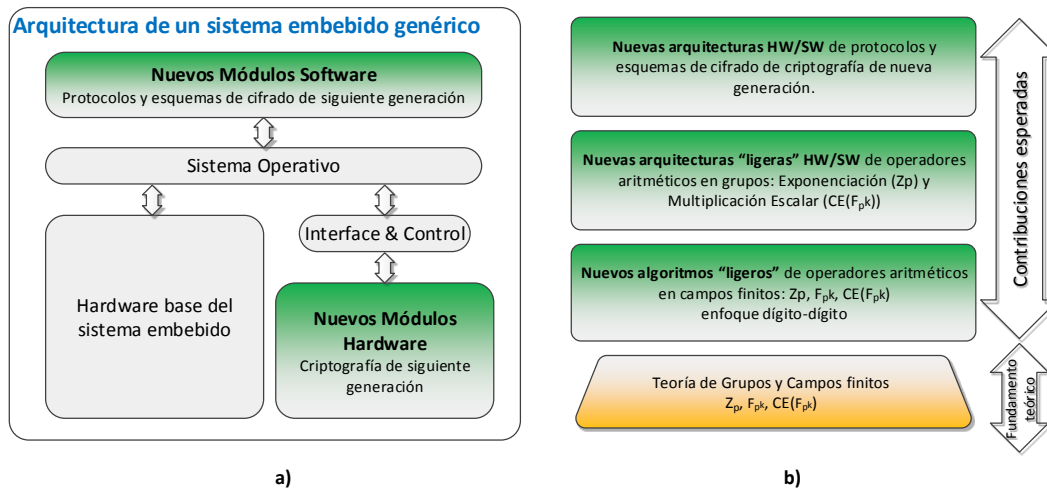
Figura 6: a) Sistema embebido con componentes Hardware/Software. b) Módulos de operadores, algoritmos, esquemas y arquitecturas de criptografía asimétrica ligera de siguiente generación que pueden incorporarse en a).
