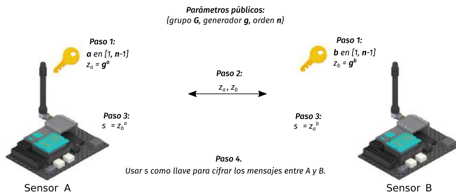
Figura 7: Establecimiento de llaves entre dos nodos sensores (sistemas embebidos). Note que el par de llaves \{a, z_a\} o \{b, z_b\} puede también ser usado en el cifrado asimétrico o la generación de firmas digitales.
