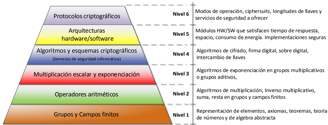
Figura 1: Distintos niveles de abstracción de mecanismos de seguridad informática basados en criptografía asimétrica.
