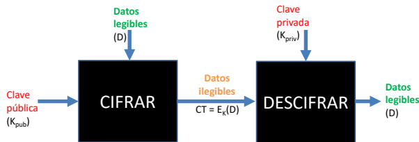
Figura 2: Procesos de cifrado (convertir texto legible a ilegible) y descifrado (convertir el texto ilegible del cifrado a texto legible nuevamente).
