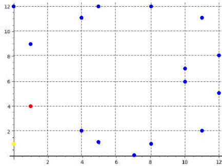
Figura 4: Ejemplo de una curva elíptica dada por la ecuación y^2 = x^3 + x + 1 \pmod{13} .
