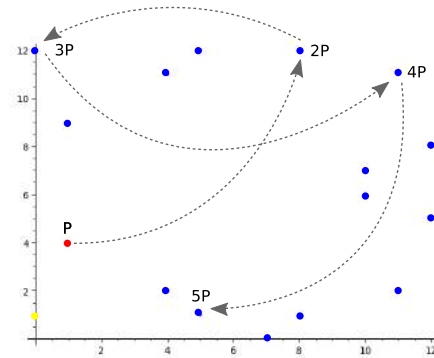
Figura 5: Comportamiento de un generador en un grupo de curva elíptica.
