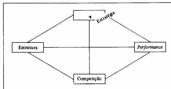
Figura 1 Modelo ampliado de Chandler
