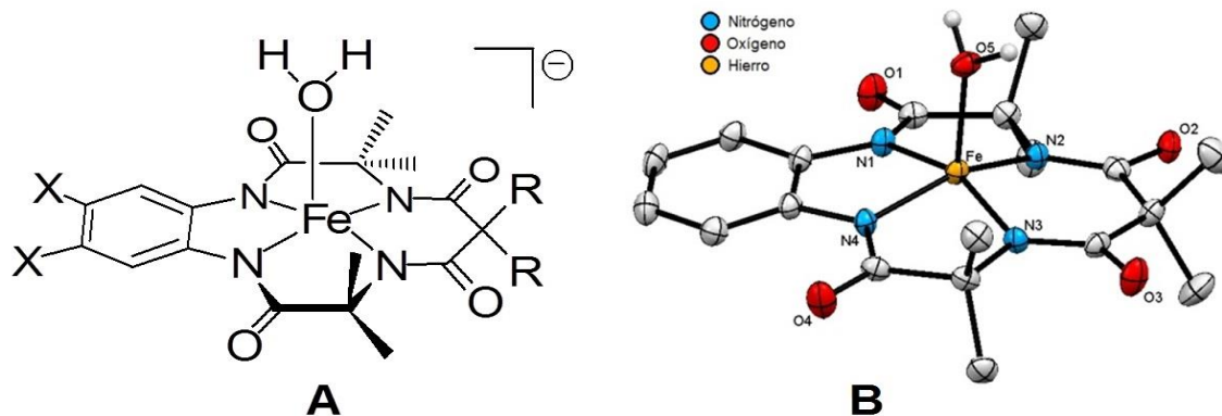
Figura 4. (A) Complejos \text{Fe}^{\text{III}} -TAMLs y (B) Estructura de Rayos-X de la parte aniónica del complejo Fe-TAML con \text{X} = \text{H} y \text{R} = \text{CH}_3 (los átomos de hidrógeno no son mostrados para claridad).
