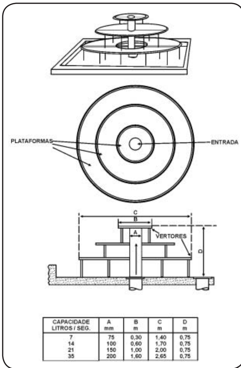
Figura 49 — Aerador de cascata
