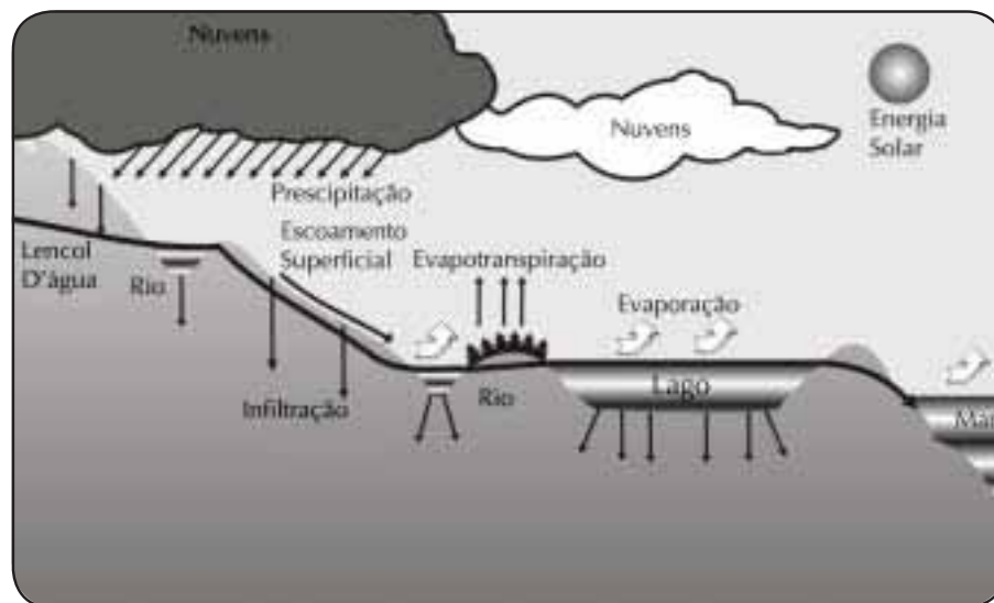
Figura 5 — Ciclo hidrológico
