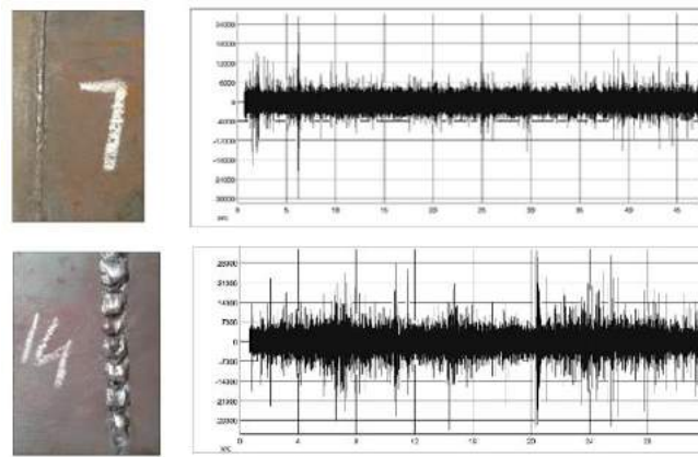
Figura 3. 5. Comparación entre un espectrograma asociado a una buena soldadura (arriba) y uno asociado a un defecto de exceso de soldadura (abajo) (Sumesh, Rameshkumar, Mohandas, & Shyam Babu, 2015)
