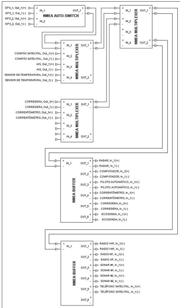
Figura 1. Interconexión entre equipos electrónicos de un barco atunero.
