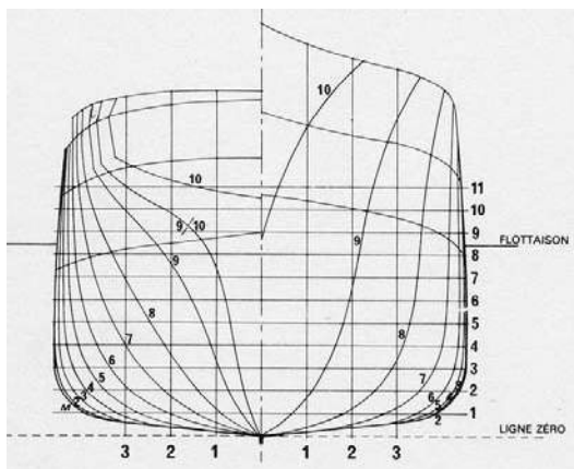
Comparación de plano de formas de un barco y plano de formas de una viga de la plataforma de la Ópera de Sydney.
