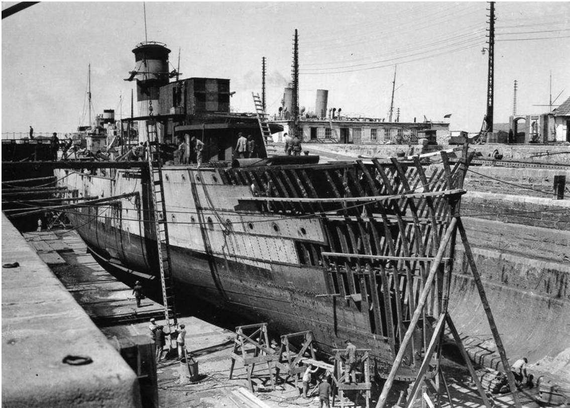
Construcción del forro y del armazón de un barco.
