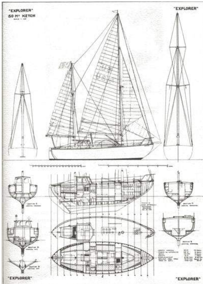
Plano de un modelo de barco diseñado por el padre de Jørn Utzon en Dinamarca.
