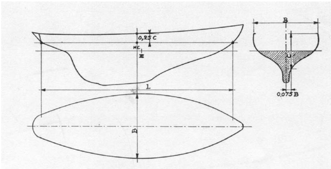
Plano de un casco de barco.
