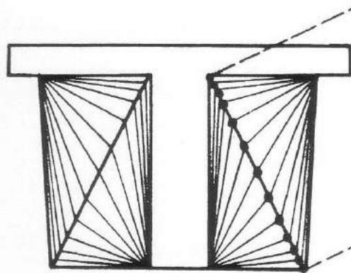
Comparación de plano de formas de un barco y plano de formas de una viga de la plataforma de la Ópera de Sydney.
