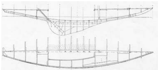
Velero de regata de mar.
