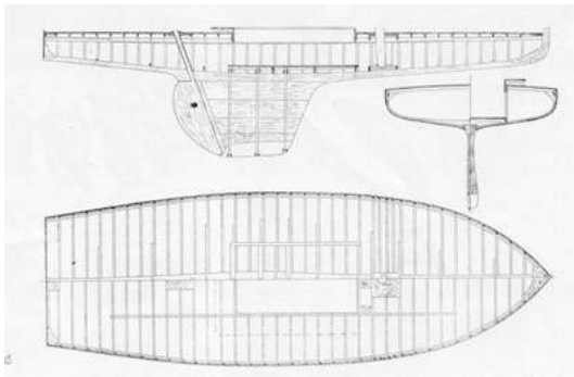
Velero de regata de río.
