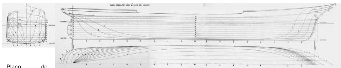
Plano de formas de un buque.
