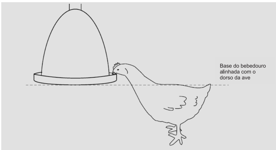
Figura 7. Diagrama de ajuste de bebedouros tipo pendular (Agrocerec Ross, 2004)
