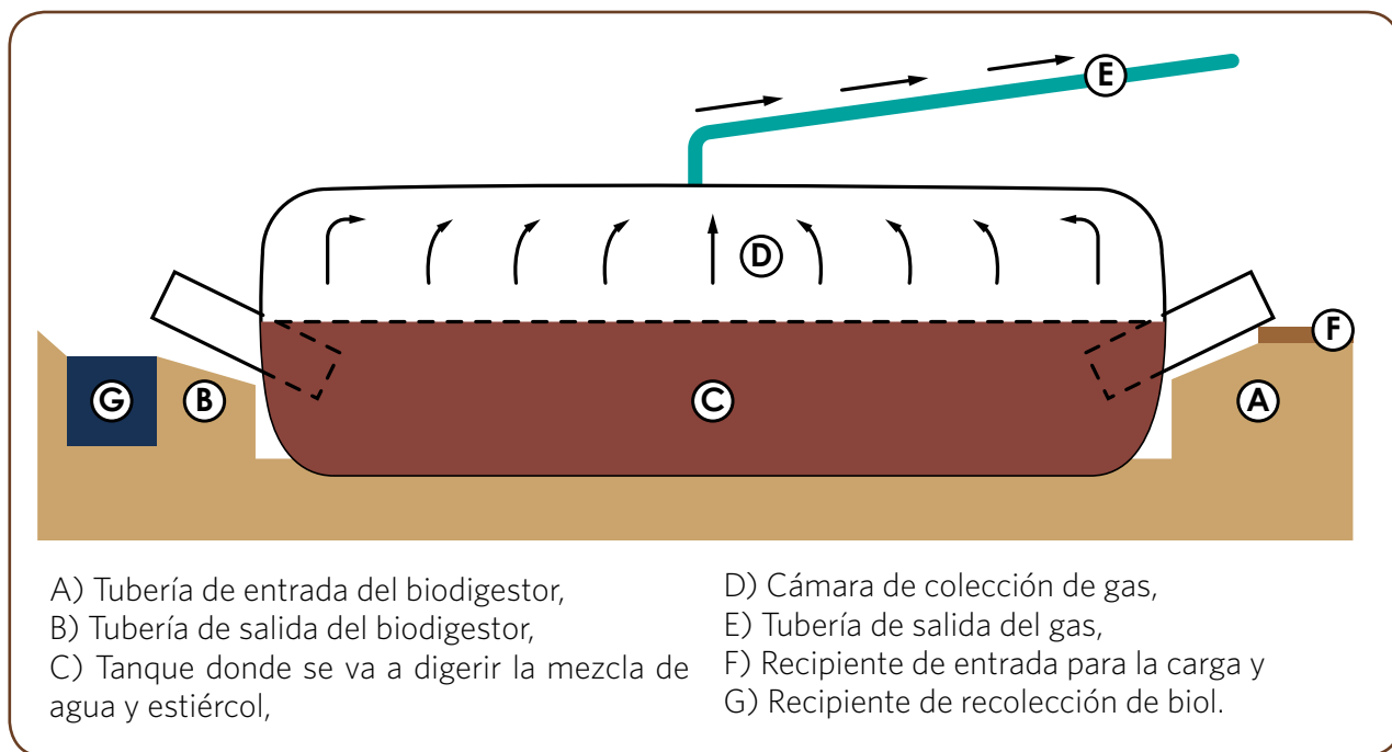
Figura 6. Partes y esquema de funcionamiento de un biodigestor tubular
