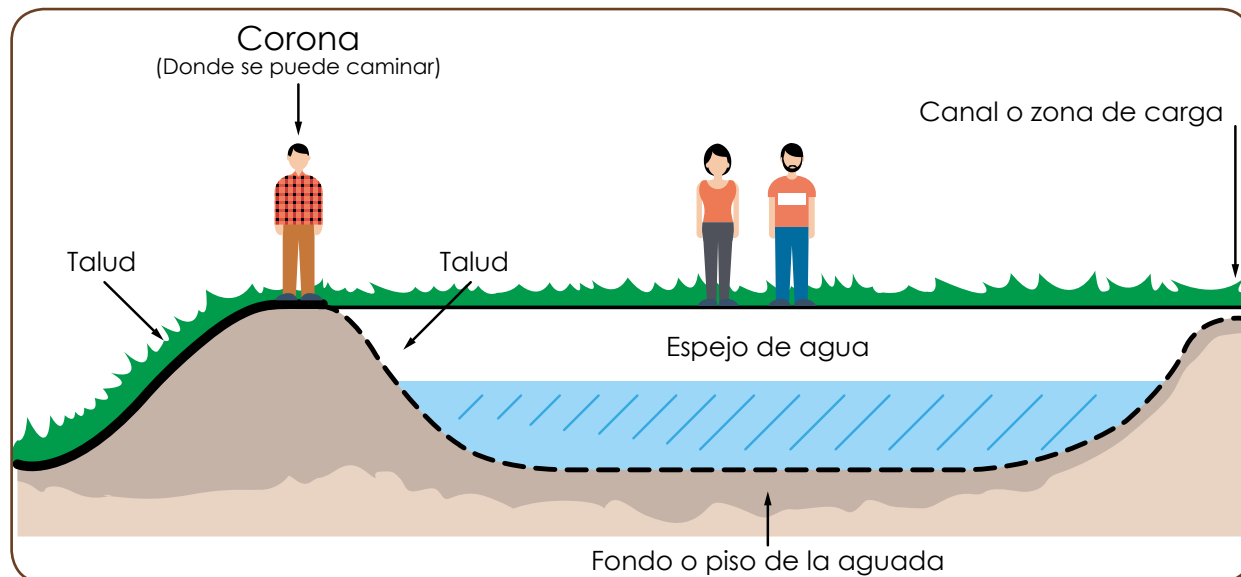
Figura 3. Partes de una aguada mejorada
