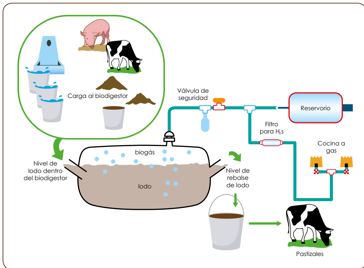
Figura 5. Sistema de un biodigestor
