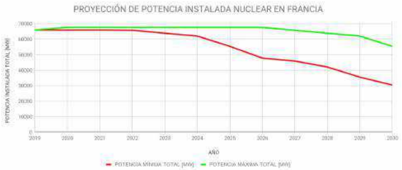
Gráfico N° 26: Proyección de potencia instalada nuclear en Francia
