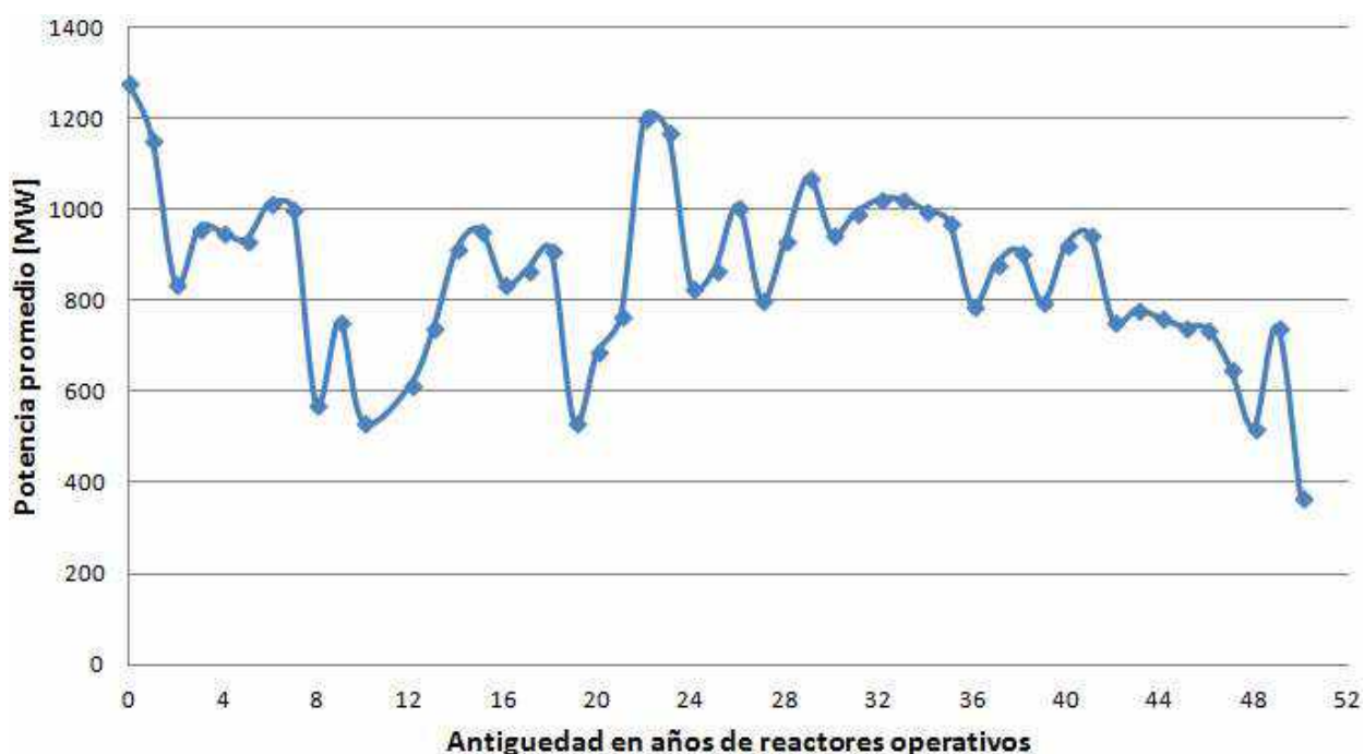
Gráfico N° 8: Potencia promedio de reactores según su antigüedad [PRIS-IAEA]
