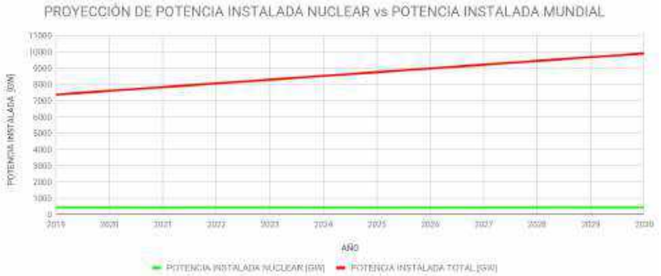
Gráfico N° 70: Proyección de potencia instalada nuclear vs potencia instalada total mundial
