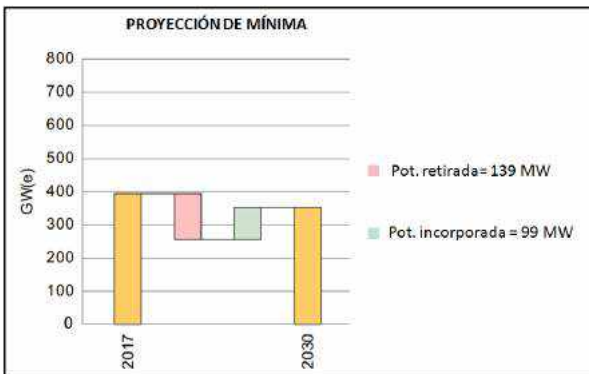
Gráfico N° 60: Proyección de mínima potencia instalada nuclear realizada por OIEA
