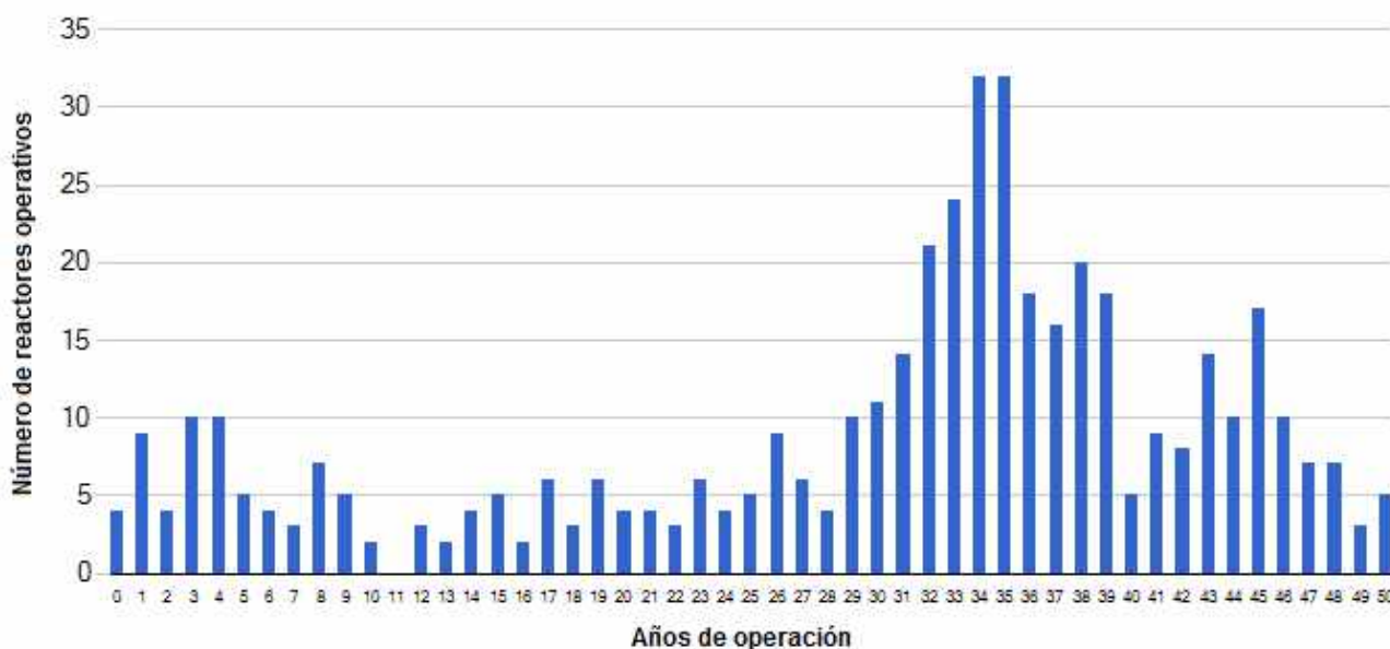
Gráfico N° 7: Cantidad de reactores operativos según antigüedad [PRIS-IAEA]
