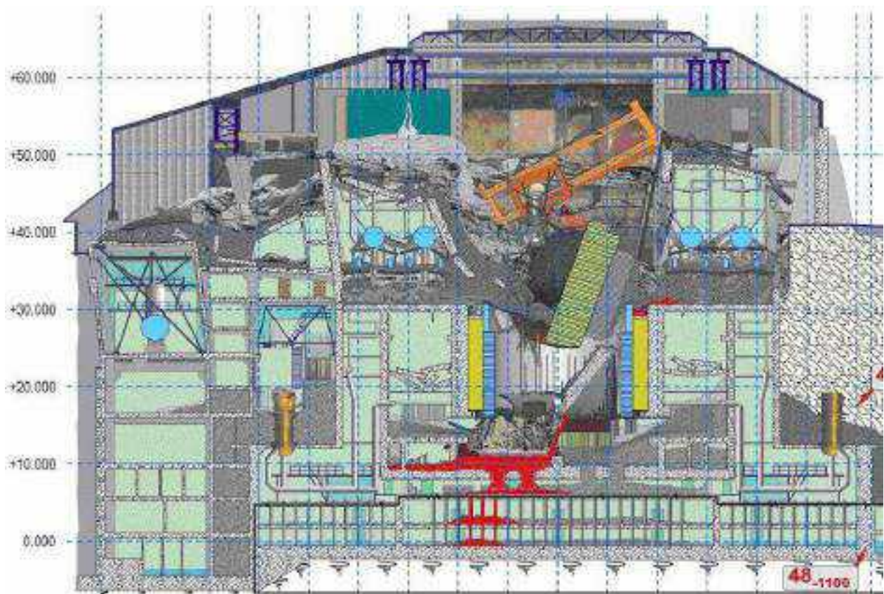
Figura N°2: Corte del Nuevo Sarcófago Seguro construido sobre la Unidad N°4 de Chernobyl
