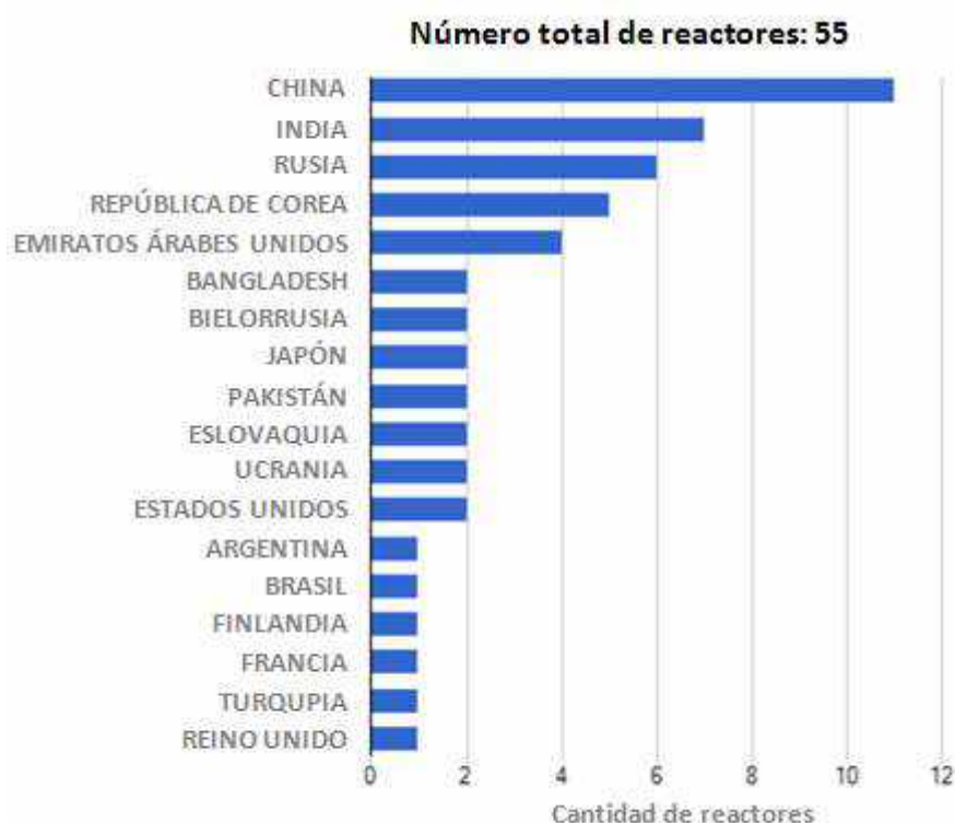
Gráfico N° 9: Reactores nucleares en construcción por país a enero de 2019 [PRIS-IAEA]
