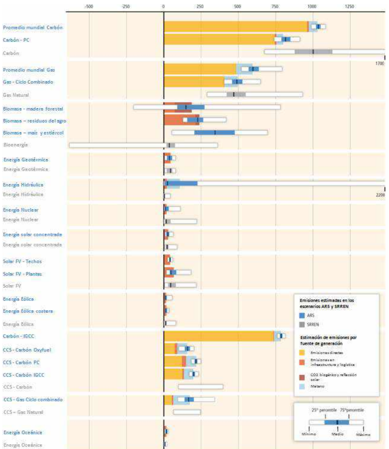
Figura N°21: Emisiones de CO 2 por tecnología [15]
