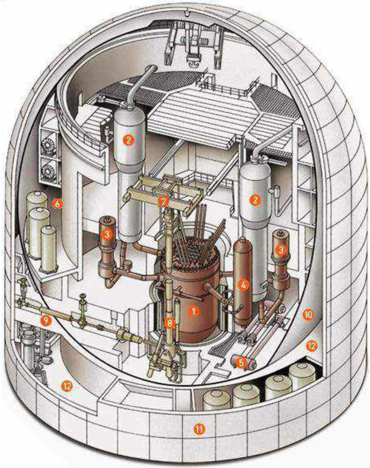
Figura N°9: Edificio del reactor de la Central Nuclear Atucha I
