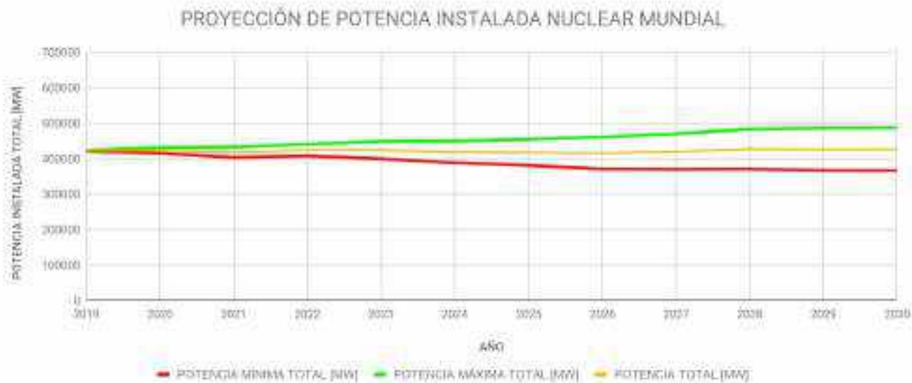
Gráfico N° 59: Proyección de potencia instalada nuclear en el mundo
