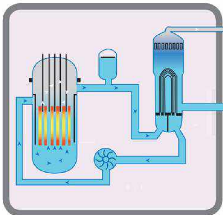
Figura N°12: Esquema de un reactor de tipo PWR
