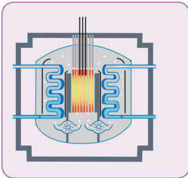
Figura N°16: Esquema de un reactor de tipo GCR
