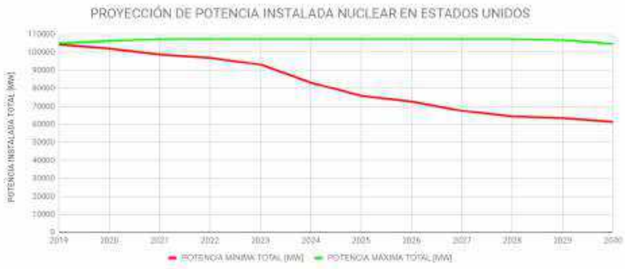
Gráfico N° 20: Proyección de potencia instalada nuclear en Estados Unidos
