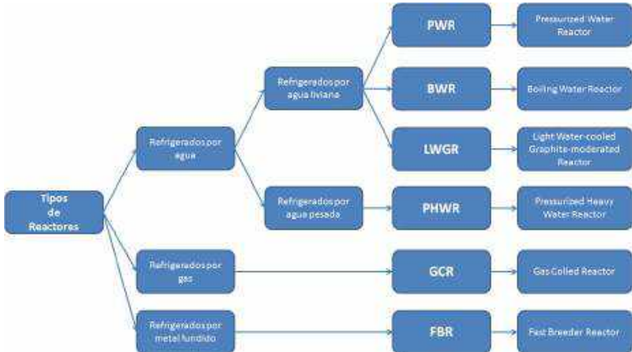
Figura N°11: Principales tecnologías de generación nuclear [Elaboración propia]
