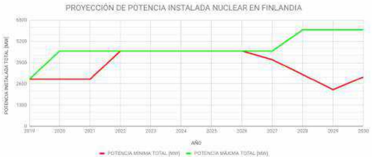
Gráfico N° 25: Proyección de potencia instalada nuclear en Finlandia
