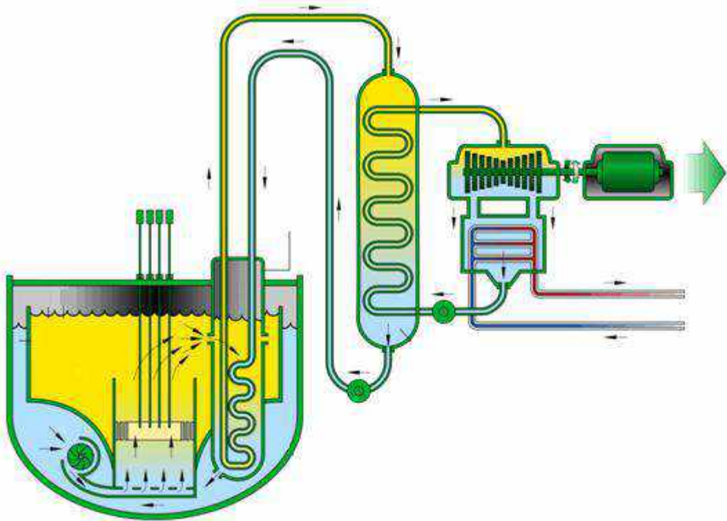
Figura N°17: Esquema de un reactor de tipo FBR
