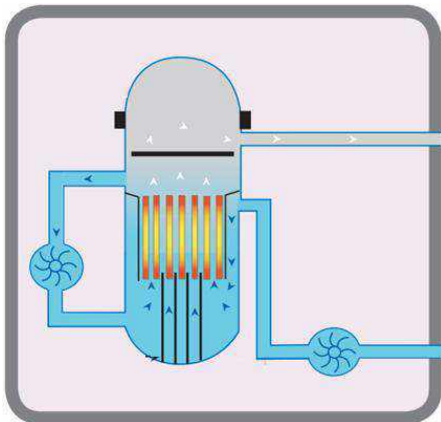
Figura N°13: Esquema de un reactor de tipo BWR
