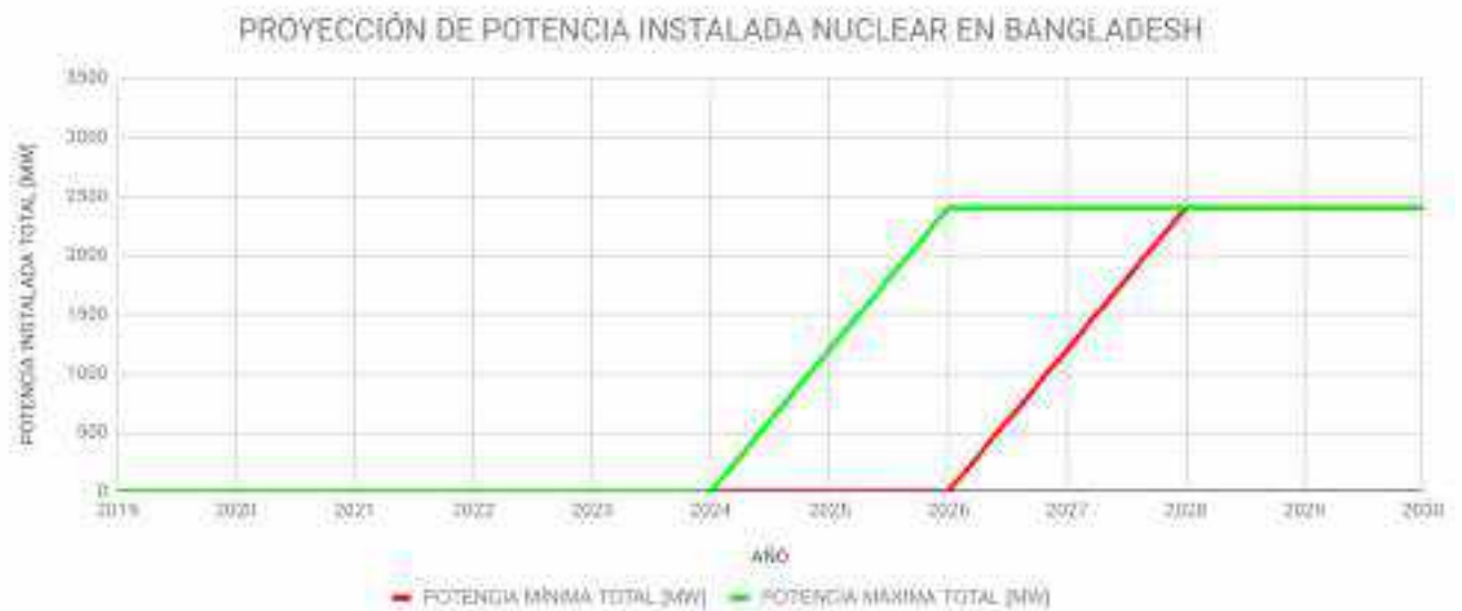
Gráfico N° 50: Proyección de potencia instalada nuclear en Bangladesh
