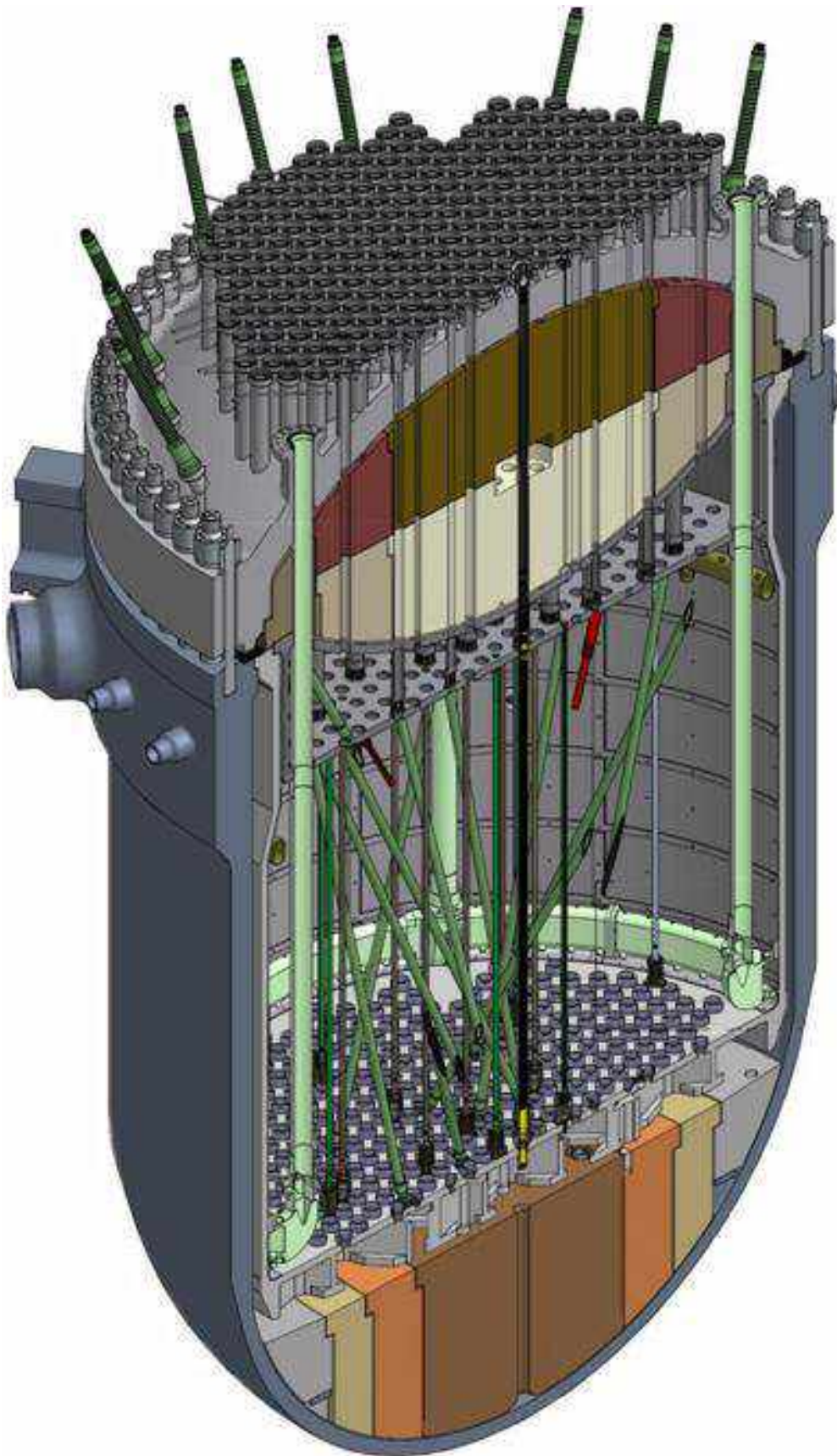
Figura N°8: Corte del recipiente de presión de Atucha II
