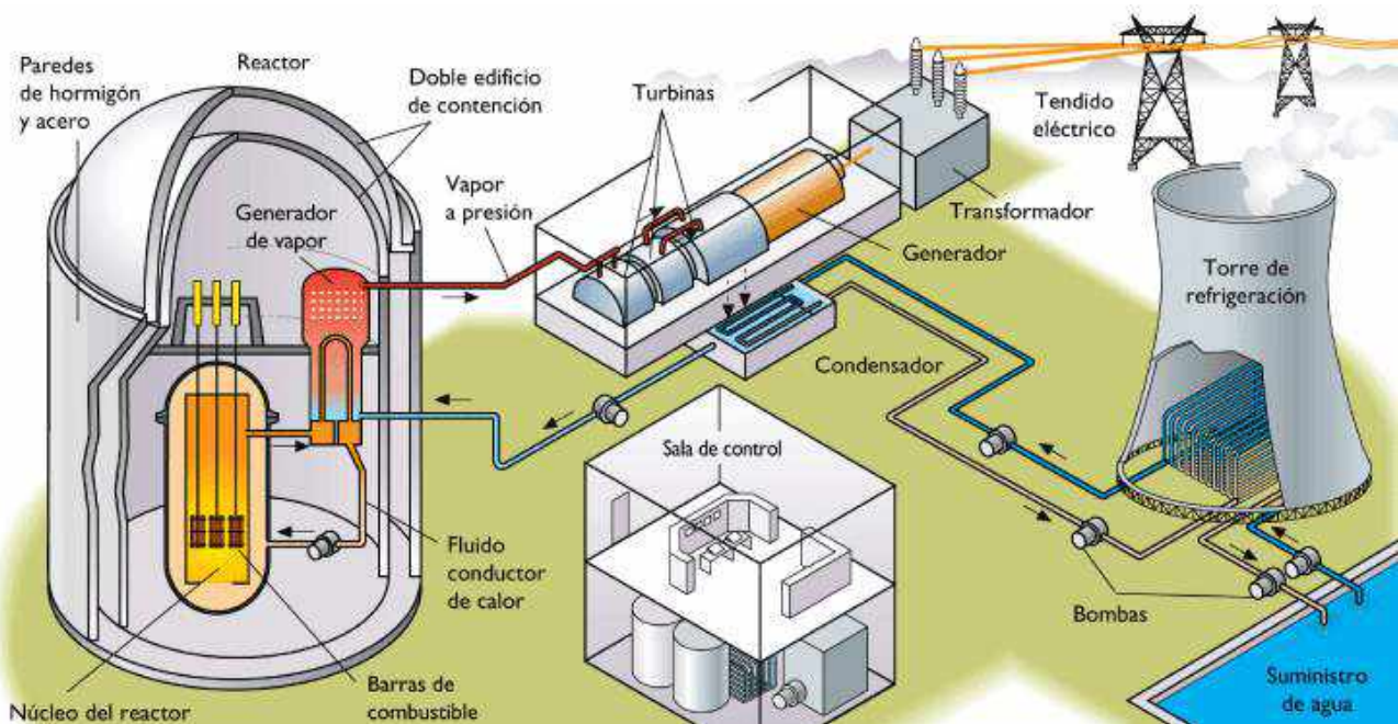
Figura N°7: Esquema de una central nuclear convencional
