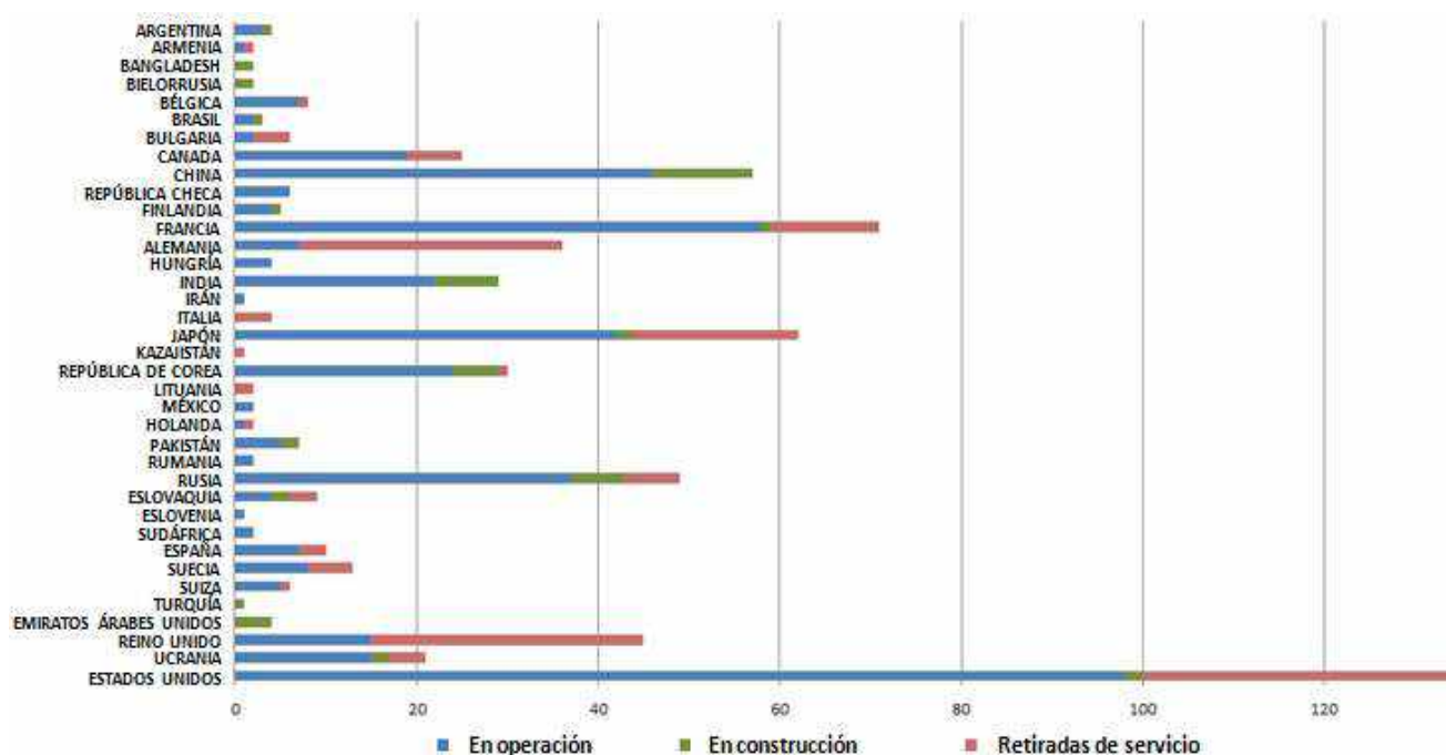
Gráfico N° 16: Centrales nucleares por país con su correspondiente estado [PRIS-IAEA]
