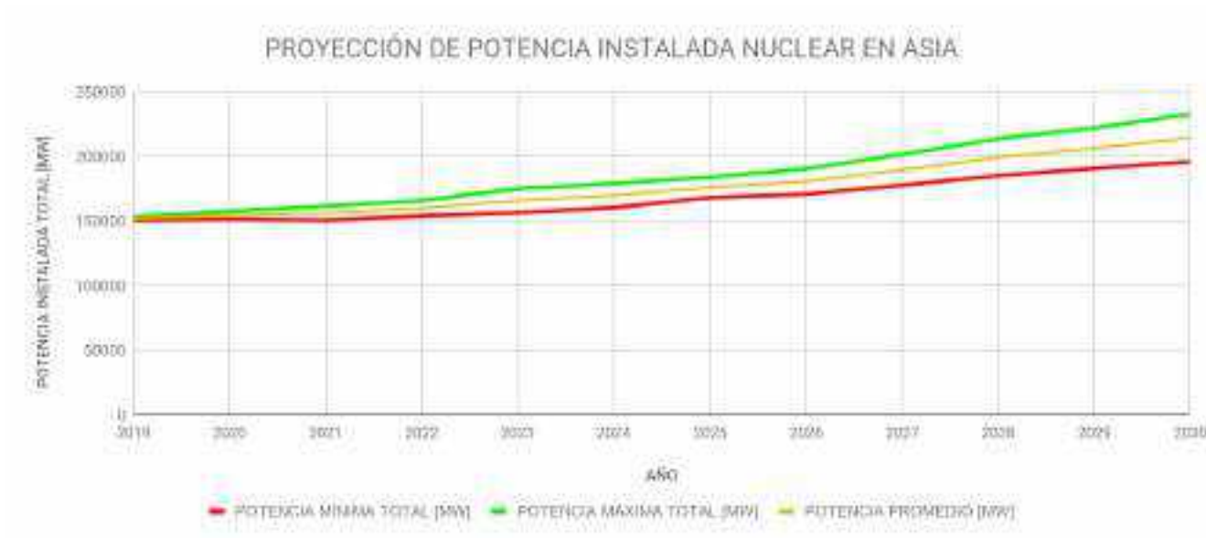
Gráfico N° 57: Proyección de potencia instalada nuclear en Asia
