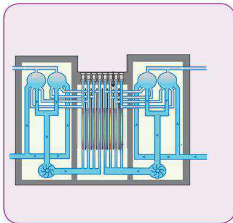
Figura N°14: Esquema de un reactor de tipo LWGR
