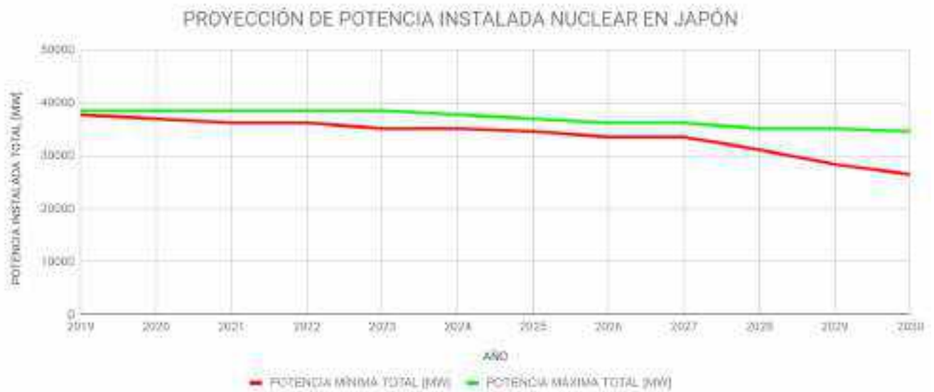
Gráfico N° 43: Proyección de potencia instalada nuclear en Japón
