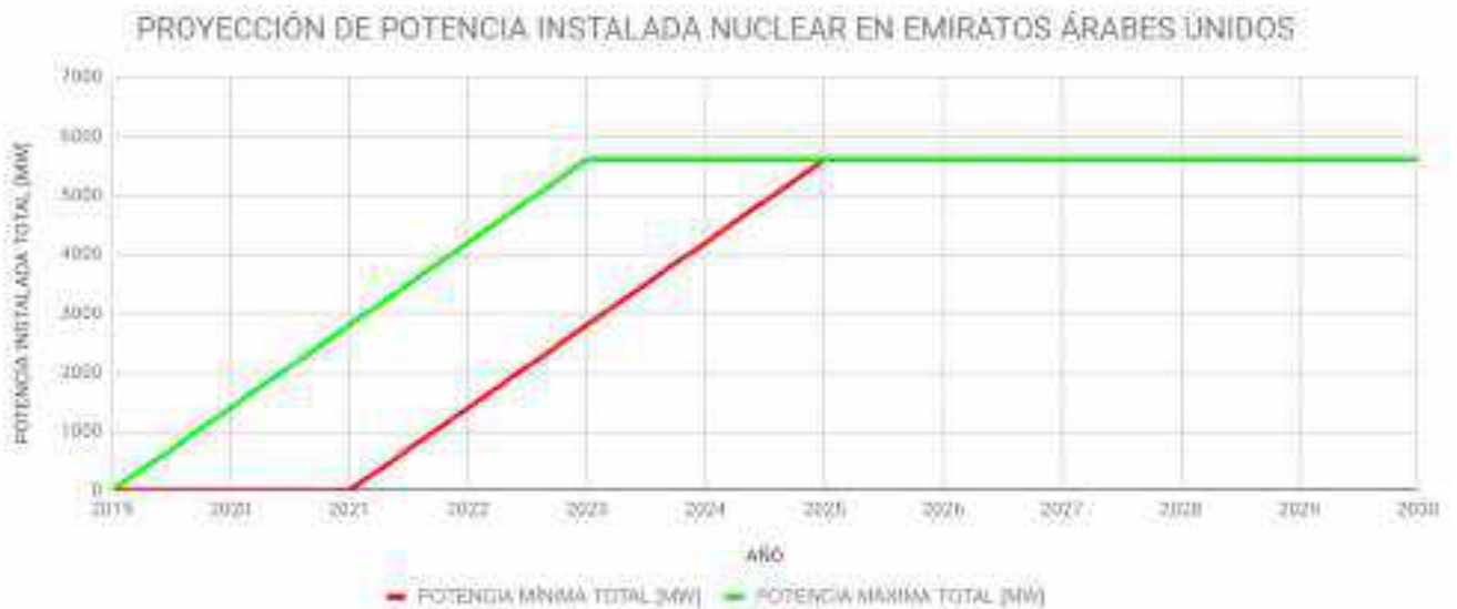
Gráfico N° 52: Proyección de potencia instalada nuclear en Emiratos Árabes Unidos
