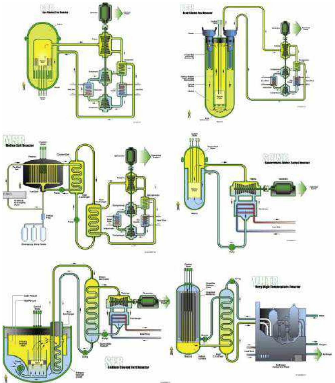
Figura N°19: Concepto de las 6 tecnologías de reactores nucleares de Generación IV
