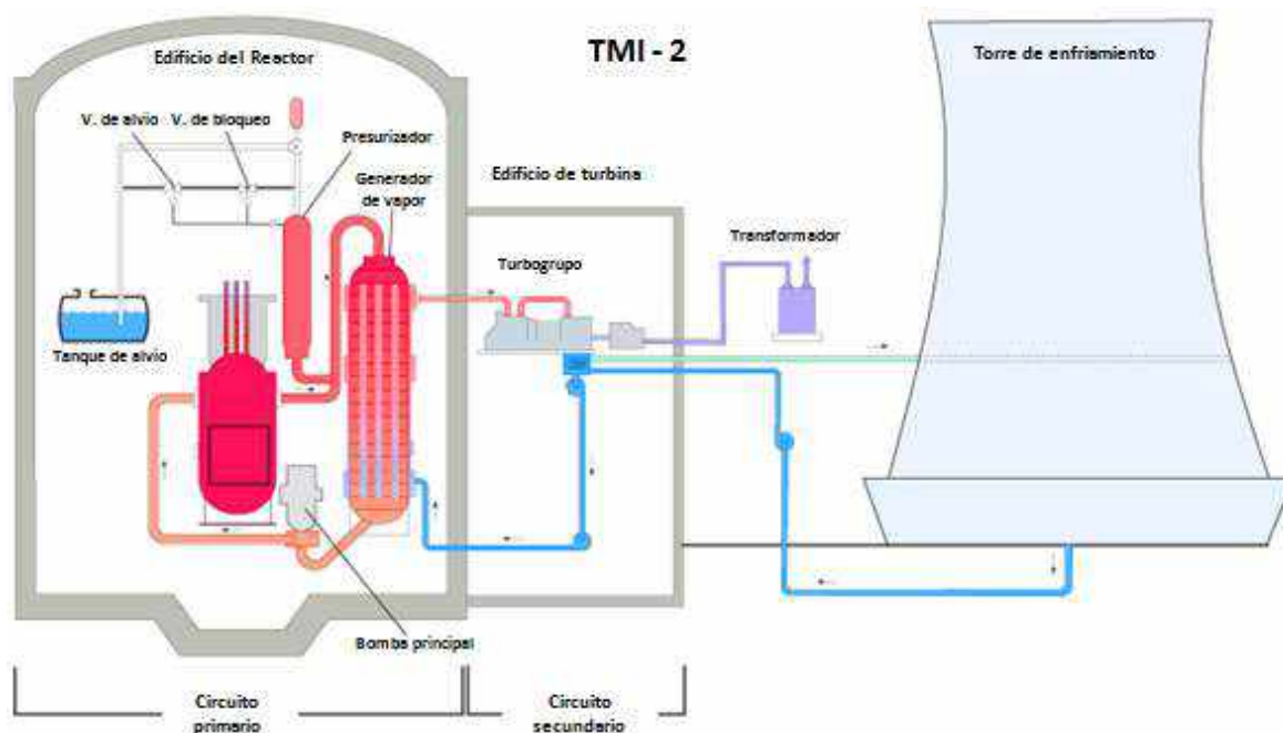
Figura N°1: Esquema simplificado del reactor de Three Mile Island - Unidad N°2
