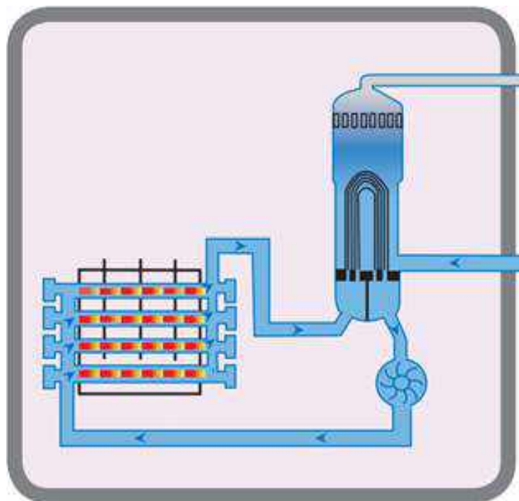
Figura N°15: Esquema de un reactor de tipo PHWR-CANDU
