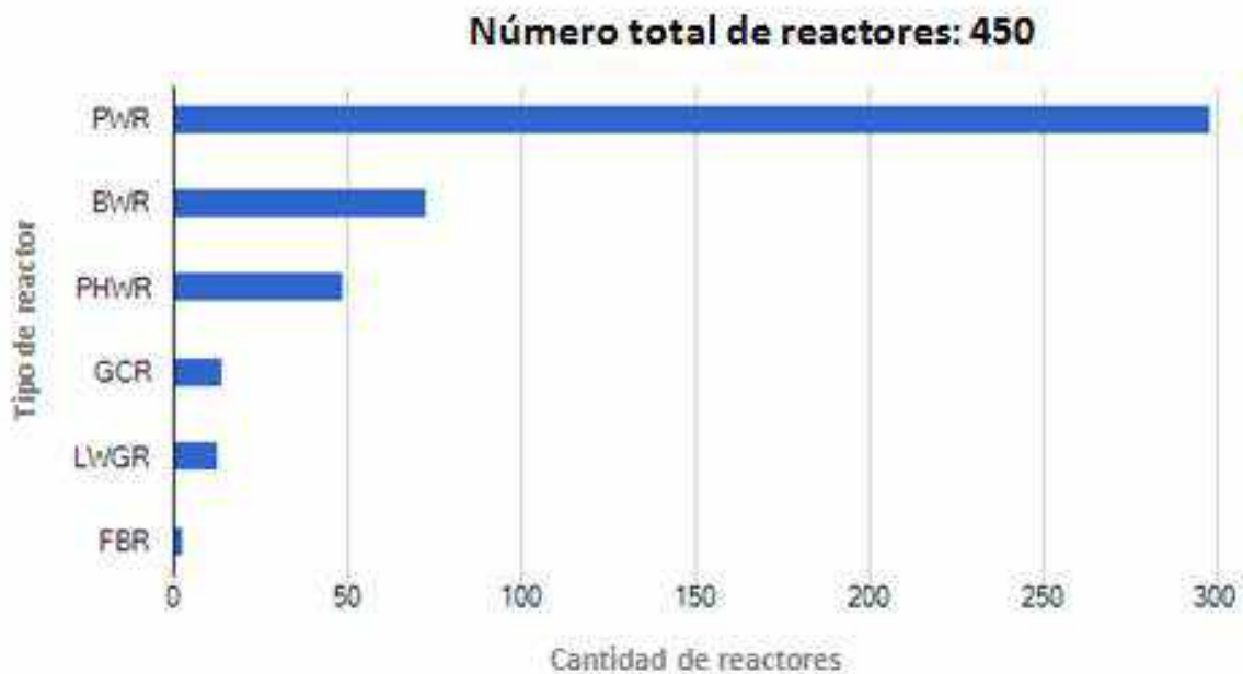
Gráfico N° 66: Cantidad de reactores en operación ordenados por tecnología [PRIS-IAEA]
