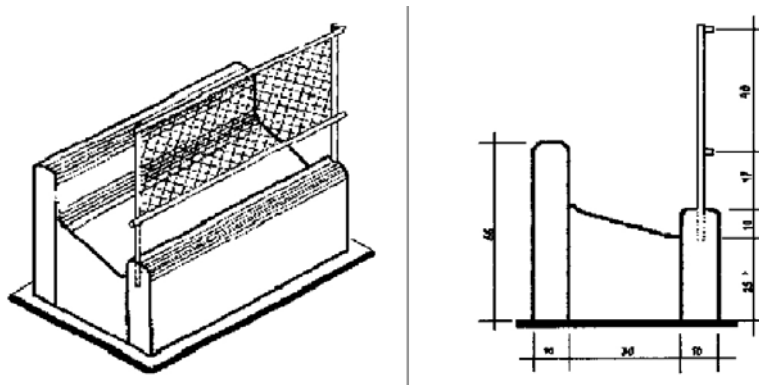
Figura 2. Vista general de un comedero y sus dimensiones
