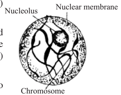
Fig. 4.15a Leptotene
