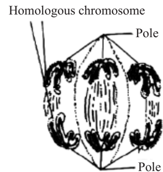
Fig. 4.15g Anaphase
