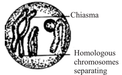
Fig. 4.15e Diakinesis
