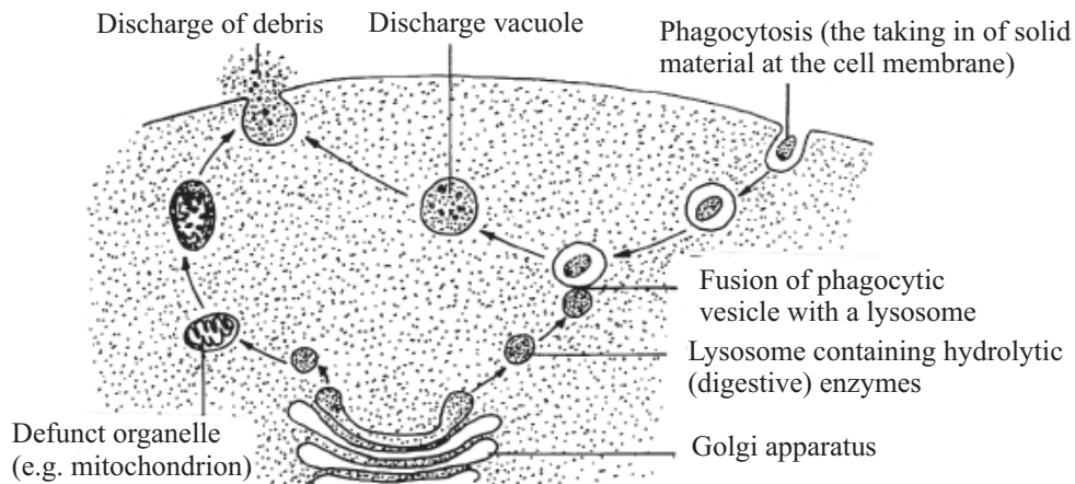
Fig. 4.9 Lysosomes
