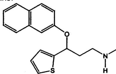
Duloxetina
