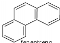
fenantreno
