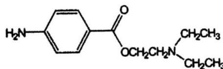
Procaina
