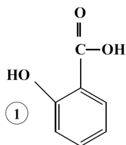
Ácido Salicílico
