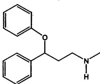
Fluoxetina
