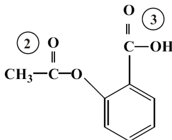
Ácido Acetilsalicílico
