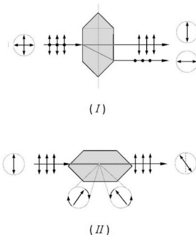
Figura 2: (I) A birrefringência linear no quartzo: o raio incidente, não polarizado, o atravessa perpendicularmente ao eixo óptico, dando origem aos raios ordinário e extraordinário, analogamente ao espato da Islândia. (II) A birrefringência circular no quartzo: o raio incidente, linearmente polarizado, atravessa o quartzo ao longo de seu eixo óptico e emerge linearmente polarizado, porém com o plano de polarização rotacionado (lei de Biot). No interior do quartzo coexistem dois modos de polarização circular, esquerdo e direito, propagando-se com velocidades distintas.
