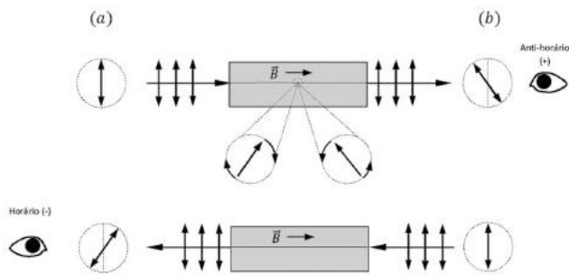
Figura 4: Ilustração de um raio de luz, inicialmente plano polarizado, propagando-se através de um material dotado de atividade óptica induzida magneticamente . No percurso de ida de (a) para (b), movendo-se no mesmo sentido em que aponta o campo magnético, sofre rotação anti-horária segundo o ponto de vista do observador em (b), que o define como esquerdo . Tomando-se a propagação em sentido inverso, movendo-se em sentido oposto ao campo magnético, um observador em (a) caracterizará a rotação como horária, segundo o seu ponto de vista. Como resultado, o plano de polarização de um mesmo raio polarizado que atravessa o meio cuja atividade óptica foi induzida magneticamente, num percurso de ida e volta, sofre rotação em dobro.
