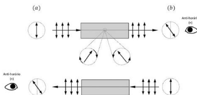
Figura 3: Ilustração de um raio de luz, inicialmente plano polarizado, propagando-se através de um fluido dotado de atividade óptica natural . No percurso de ida de (a) para (b) sofre rotação anti-horária segundo o ponto de vista do observador em (b), que identifica o meio como esquerdo . Tomando-se a propagação em sentido inverso, um observador em (a) igualmente caracterizará a rotação como anti-horária, segundo o seu ponto de vista, e o identifica como esquerdo . Como resultado, o plano de polarização de um mesmo raio polarizado que atravessa o meio opticamente ativo num percurso de ida e volta, não sofre rotação alguma. O mesmo cancelamento ocorreria se o meio opticamente ativo fosse direito .
