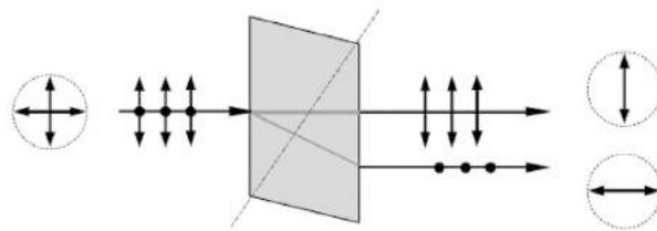
Figura 1: A birrefringência no espato da Islândia entendida a partir da hipótese da transversalidade de Fresnel: o raio incidente, não polarizado, dá origem aos raios ordinário e extraordinário de velocidades distintas, no interior do espato. Estes últimos não são capazes de formar padrões de interferência, pois correspondem a vibrações mutuamente ortogonais.
