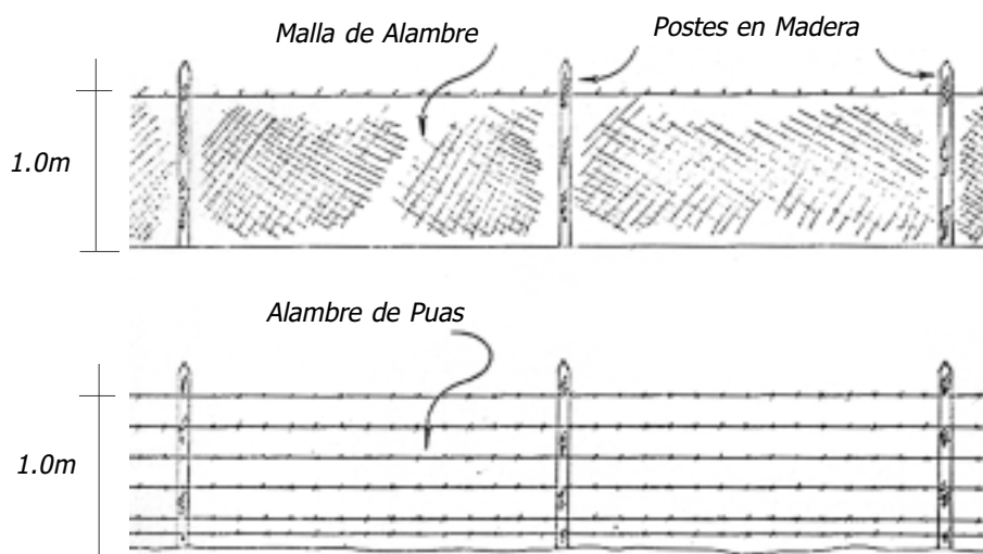
CERCAS PARA PASTOREO DE CERDOS
