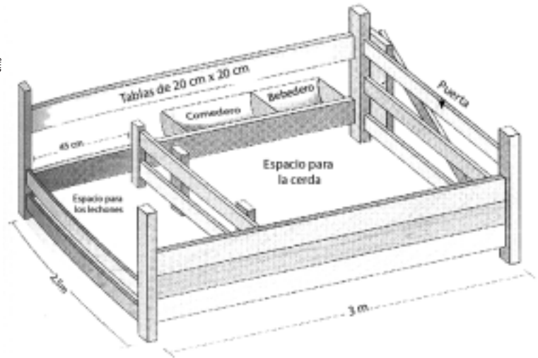
Esquema de Jaula Paritoria Individual
