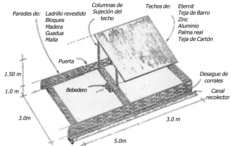
Corrales de Crecimiento y Engorde
