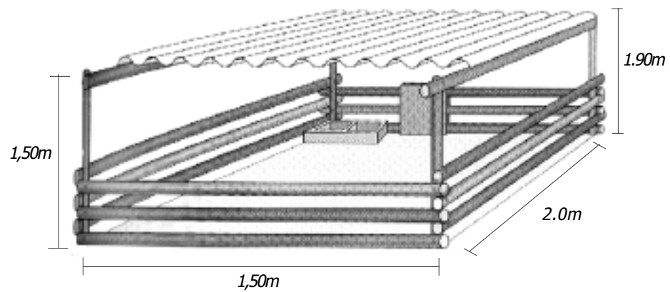
Medidas de Corral de Ceba
