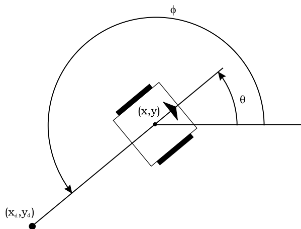
Figura 4.14: Exemplo onde o objetivo x_d e y_d encontram-se atrás do robô.
