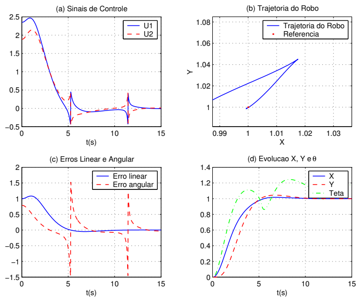
Figura 6.5: Simulação demonstrando chaveamento do sinal de controle.
