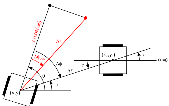
Figura 4.12: Exemplo de referência móvel em conjunto com controle de posição.
