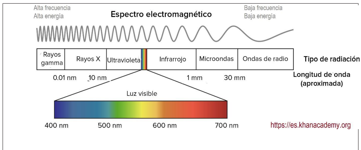
Figura 11.3. Espectro electromagnético: energía radiante desde la radiación gamma hasta las ondas de radar. Abajo, la luz blanca se descompone en un conjunto de colores llamados primarios (azul, amarillo y rojo); el verde es la combinación de los dos primeros y el naranja de los dos últimos. Fuente: https://es.khanacademy.org
