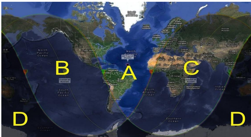
Figura 3.14. Zonas de observación del Tránsito de Mercurio 9-05-2016: A, de visibilidad total; B y C, de visibilidad parcial; en D, no es visible. Imagen, en infobservador.com
