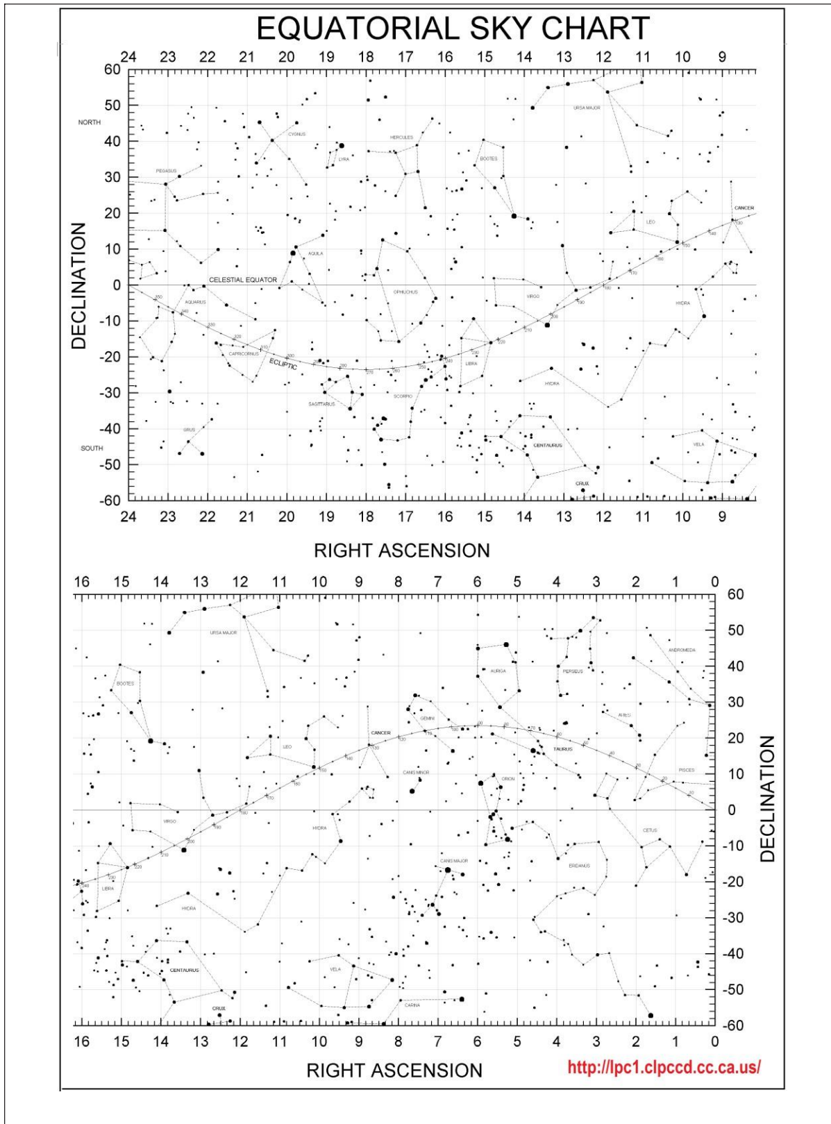
Figura 7.6 Carta Celeste Ecuatorial. http://ipc1.clpccd.cc.ca.us/
