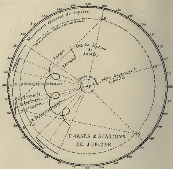
Fig. 1. Mouvement de ♃ 1.
