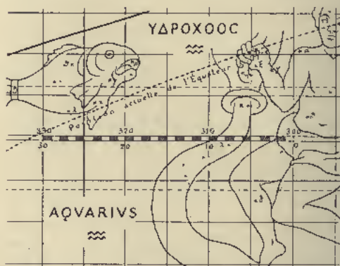
Fig. 13. Le Verseau.
