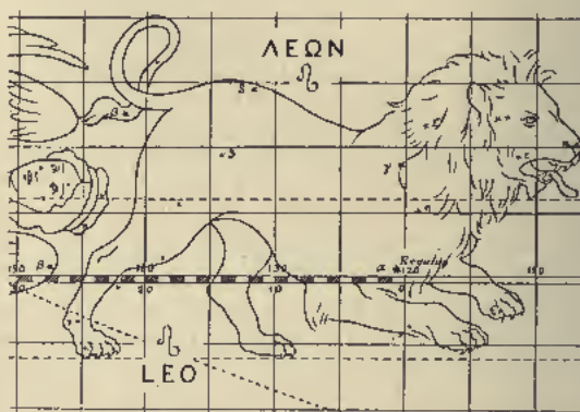
Fig. 7. Le Lion.
