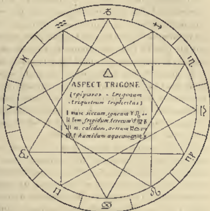
Fig. 10. Lex Trigones.
