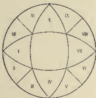
Fig. 34. Tracé circulaire.
