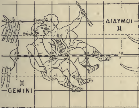
Fig. 5. Les Gémeaux.
