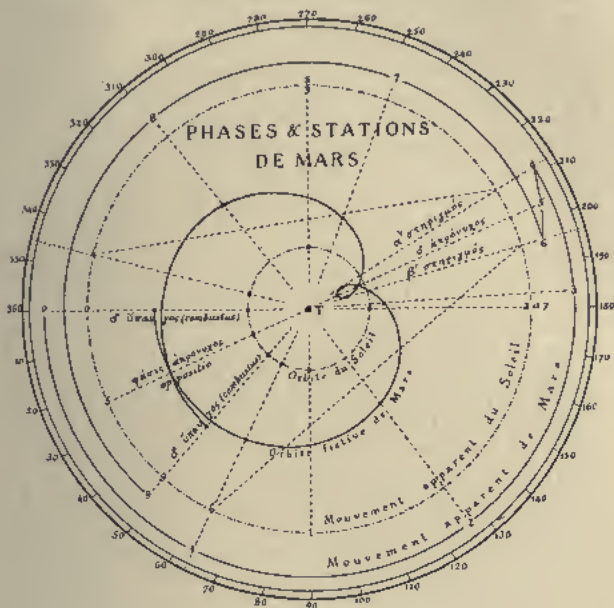
Fig. 2. Mouvement de \text{M}^1 .
