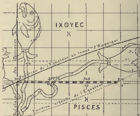
Fig. 14. Les Poissons.
