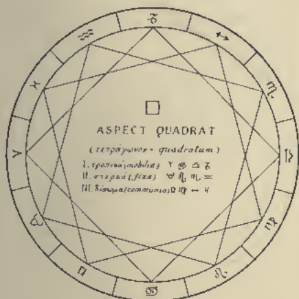
Fig. 26. Aspect quadrat.
