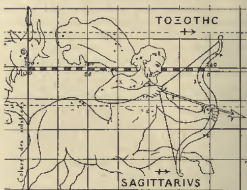
Fig. 11. Le Sagittaire.
