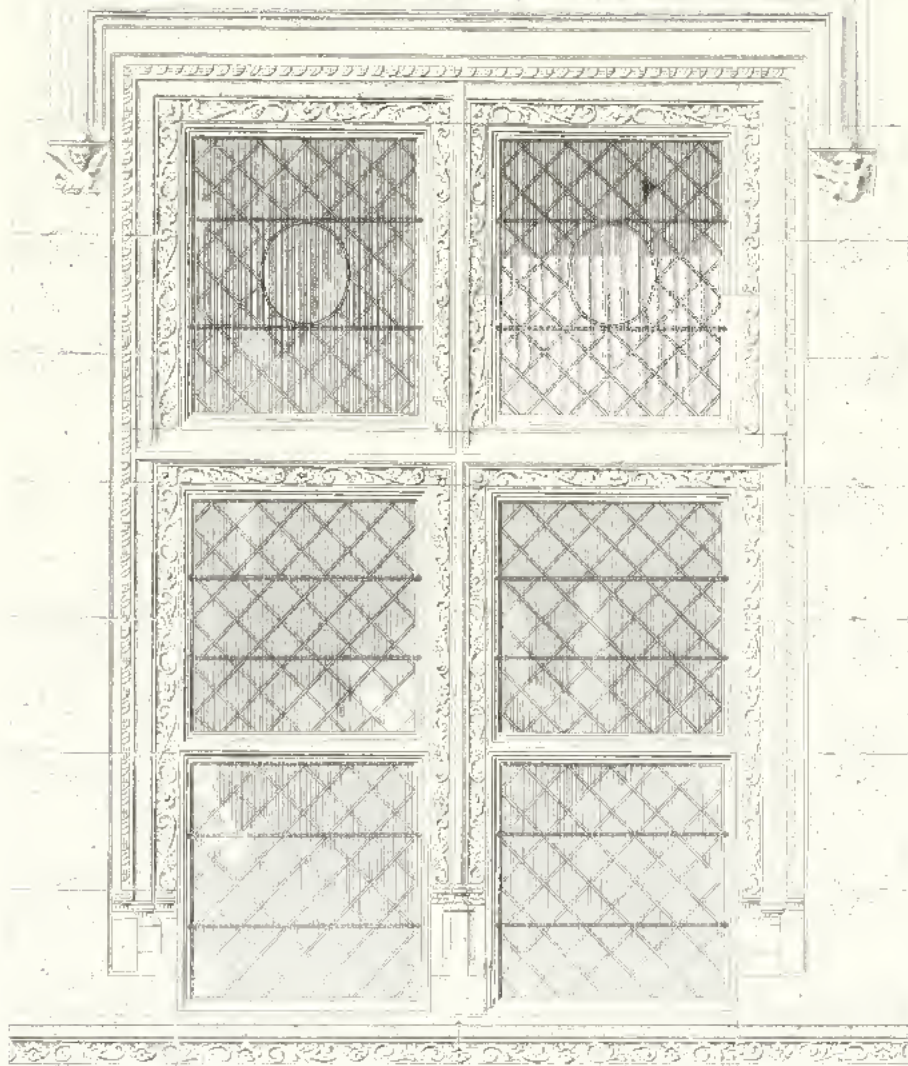
Profil de la grande croisée à six carreaux
