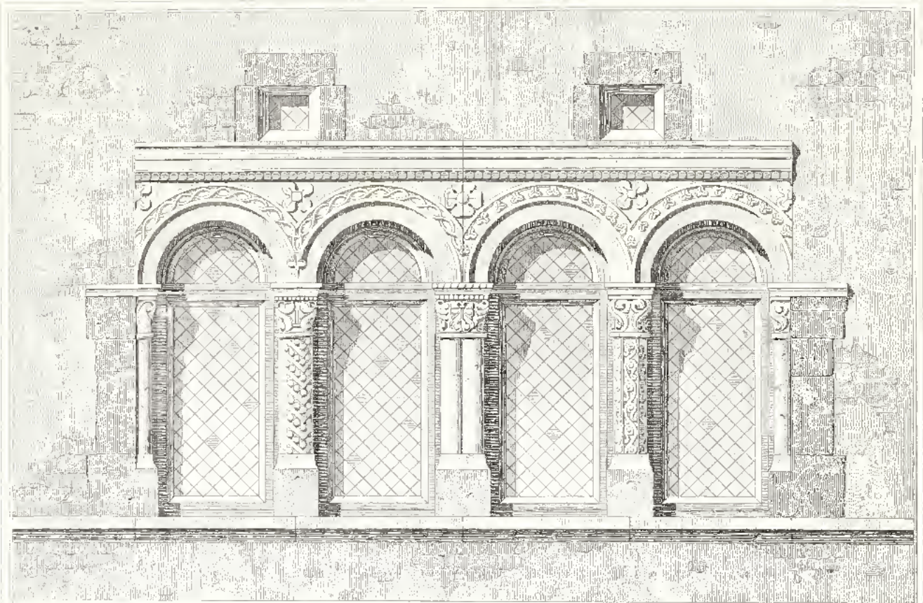
Élévation du 1 er étage de la Maison N o 2 à Cluses
