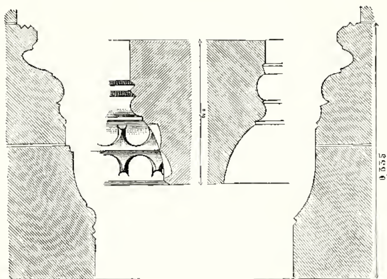
PROFILS DES BASES ET DES TAILLOIRS DES CHAPITEAUX DE LA GALERIE.
