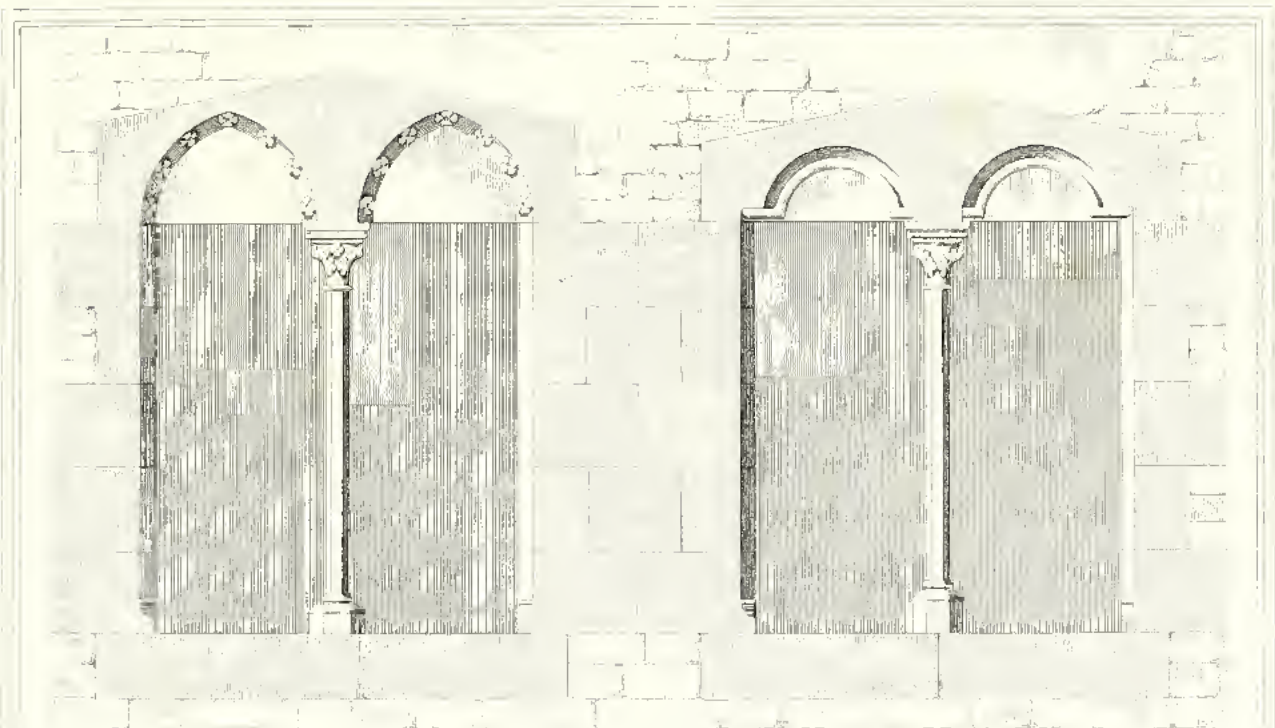
Elevée de la maison d'un Chanoine de St. Pierre à Paris
