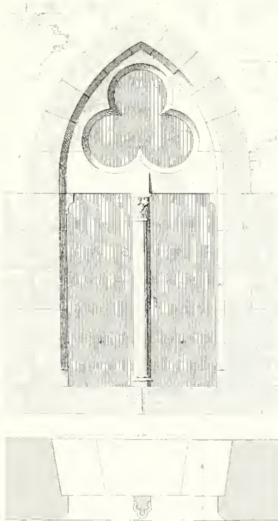
Elevée de la maison d'un Chanoine de St. Pierre à Paris
