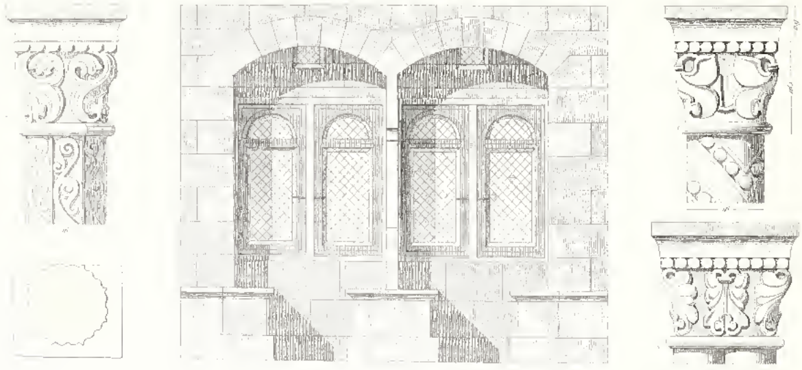
Élévation à l'intérieur à Cluses
