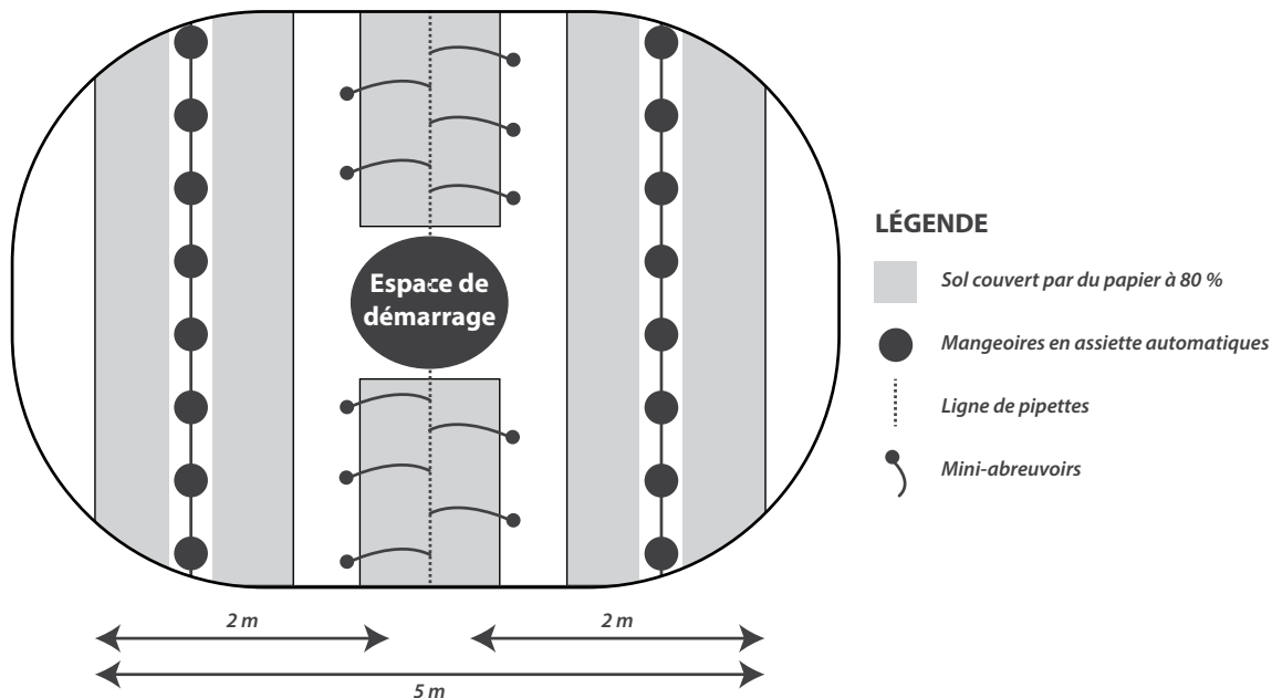
Figure 2.4 : configuration type d'un démarrage localisé (1 000 poussins).
