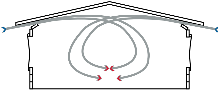
Figure 6.6 : flux d'air correct en ventilation minimale.
