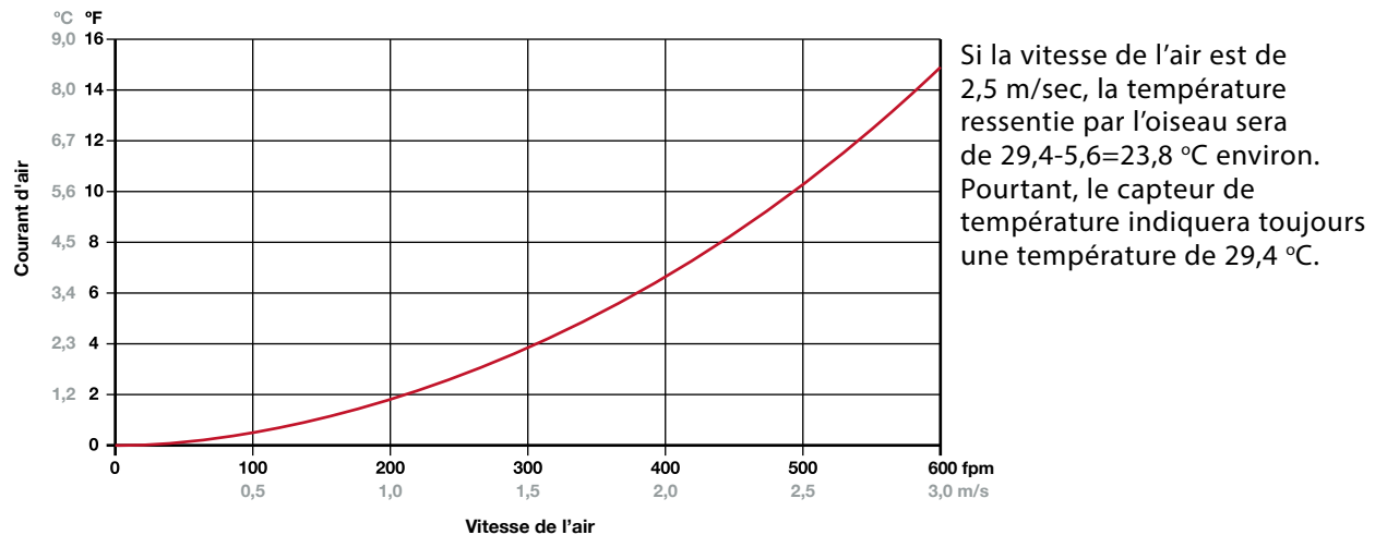
Figure 6.15 : effet de rafraîchissement théorique ressenti par un poulet de chair de 3,5 kg à une température ambiante de 29,4 °C.
