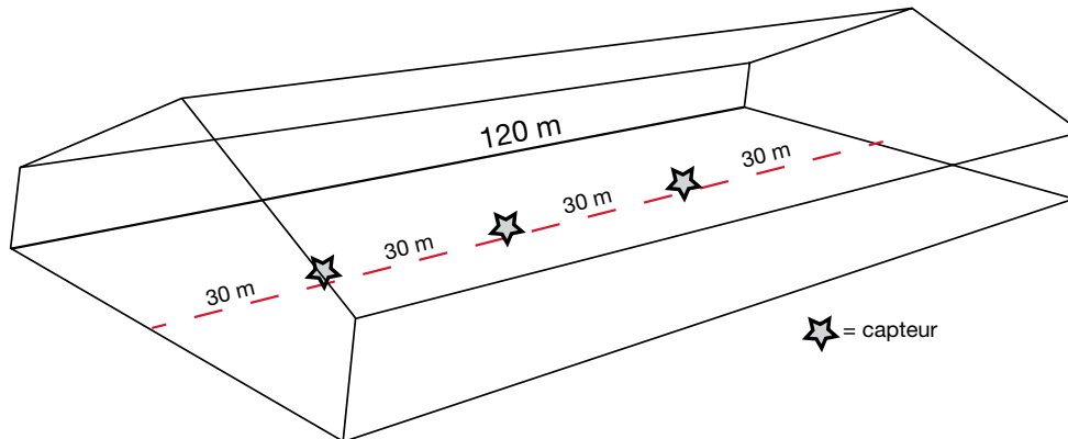
Figure 2.9 : emplacement correct des capteurs de température et d'humidité.
