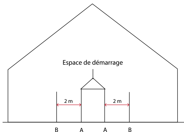
Figure 2.5 : démarrage localisé - zones en fonction des gradients de température
