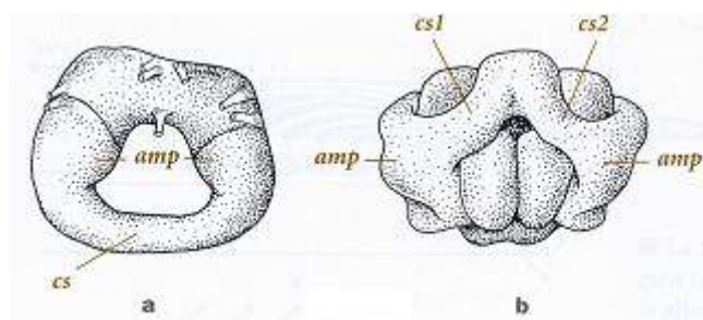
Figure 3. Canaux semi-circulaires dans l'oreille (a) chez les myxines et (b) les vertébrés.
