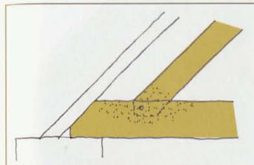
1. Avant – L'assemblage arbalétrier / entrait ne remplit plus sa fonction vu l'état de dégradation de la mortaise.
