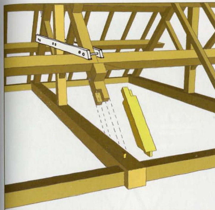
Variante d'intervention, avec remplacement du pied d'arbalétrier par une enture à bois debout dans l'arbalétrier et par tenon bloqué dans la mortaise de l'entrait. Une pièce moisée reconstitue la triangulation de la ferme pendant l'intervention.
