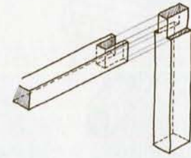
Assemblage à enfourchement.
