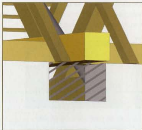
7. Le nouvel entrait est repositionné à l'aide du même Tirfor® puis la maçonnerie est reconstituée.
