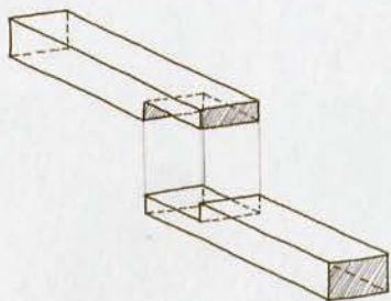
Enture à mi-bois.
