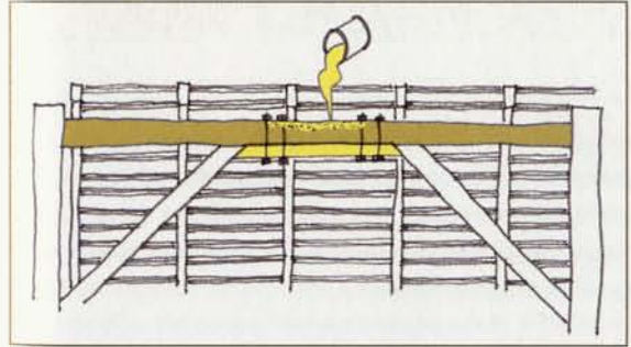
2. Après – Après avoir mis en place une pièce de renfort boulonnée, on reconstitue avec de la résine la partie de bois dégradée qui a été retirée.
