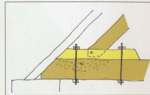
2. Après – La pièce de raccord, boulonnée sur l'entrait, recevra le pied de l'arbalétrier par un assemblage à tenon et mortaise.
