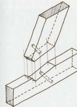
Embrèvement en about (bissectrice de l'angle d'un pied d'arbalétrier).
