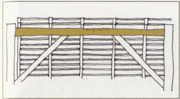
1. Avant – Seul le tiers supérieur de la panne est détérioré.
