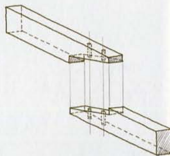
Enture en sifflet désaboté (principalement pour les fâtiages et les sablières contreventés).
