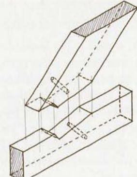
Embrèvement en décalé (d'un pied d'arbalétrier).
