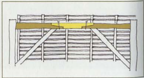
2. Après – La partie atteinte est remplacée par une pièce de bois neuve assemblée aux parties conservées par une enture à sifflet et chevillage.
