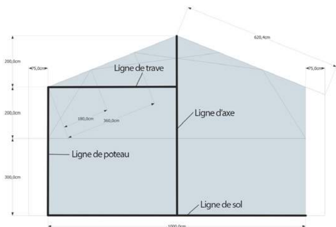
CHARPENTE 10 m
