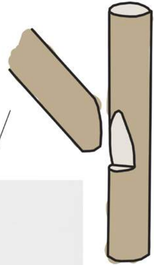
EMBRÈVEMENT D'UNE JAMBE DE FORCE SUR UN POTEAU
