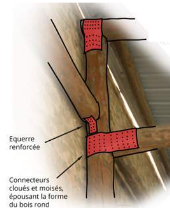
Connecteurs métalliques pour bois ronds.
