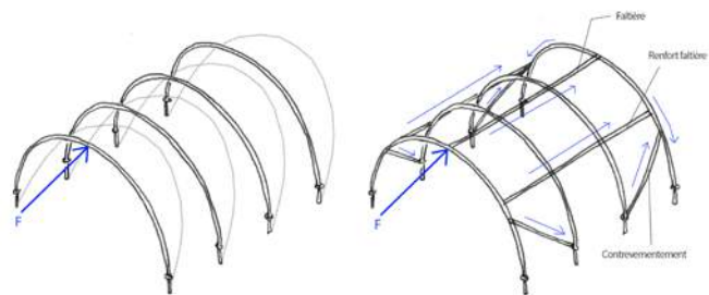
△ Exemple de fonctionnement des contreventements pour une serre.
