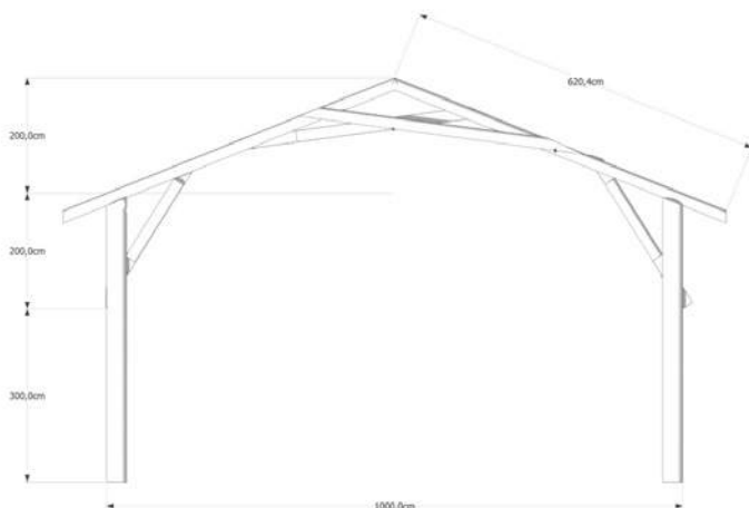
CHARPENTE 10 m
