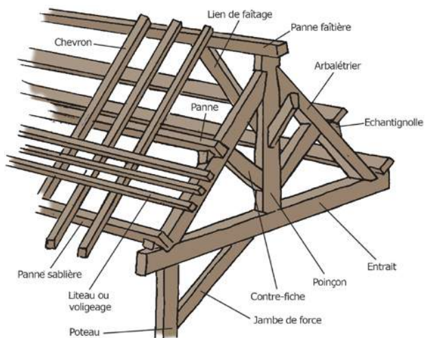
▲ Les composants d'une charpente
