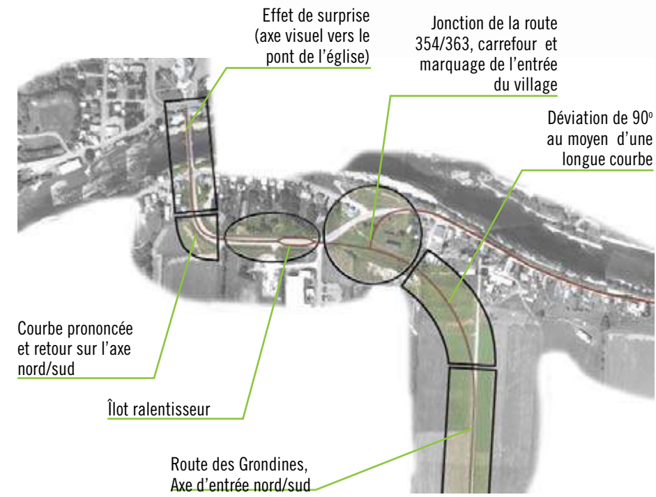
L'aménagement de la route 354 à Saint-Casimir a pour but de marquer l'entrée du village et de faire diminuer la vitesse de transit des automobilistes.
