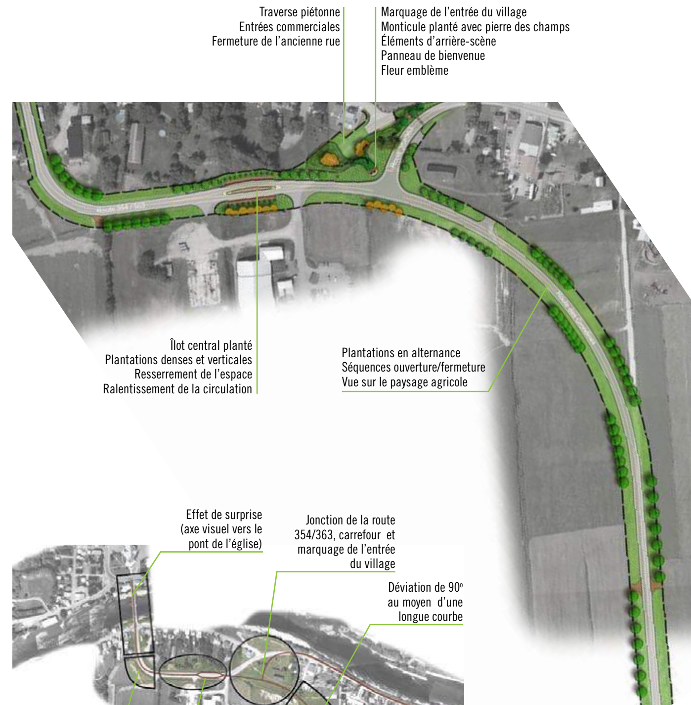
L'aménagement de la route 354 à Saint-Casimir a pour but de marquer l'entrée du village et de faire diminuer la vitesse de transit des automobilistes.
