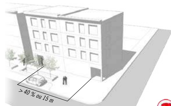
Aucun mur aveugle de plus de 40 % de la façade ou de plus de 15 m le long d'un trottoir
