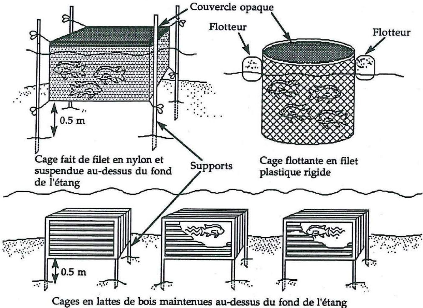
Figure 1: Exemples de cages faites de matériel divers positionnées sur ou au-dessus du fond.
