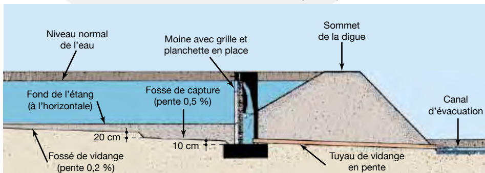
Figure 74. Coupe transversale d'un étang au niveau du fossé de vidange.
