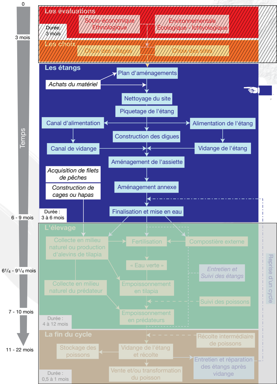
Figure 47. Mise en place d'étangs piscicoles : 3. Les étangs.
