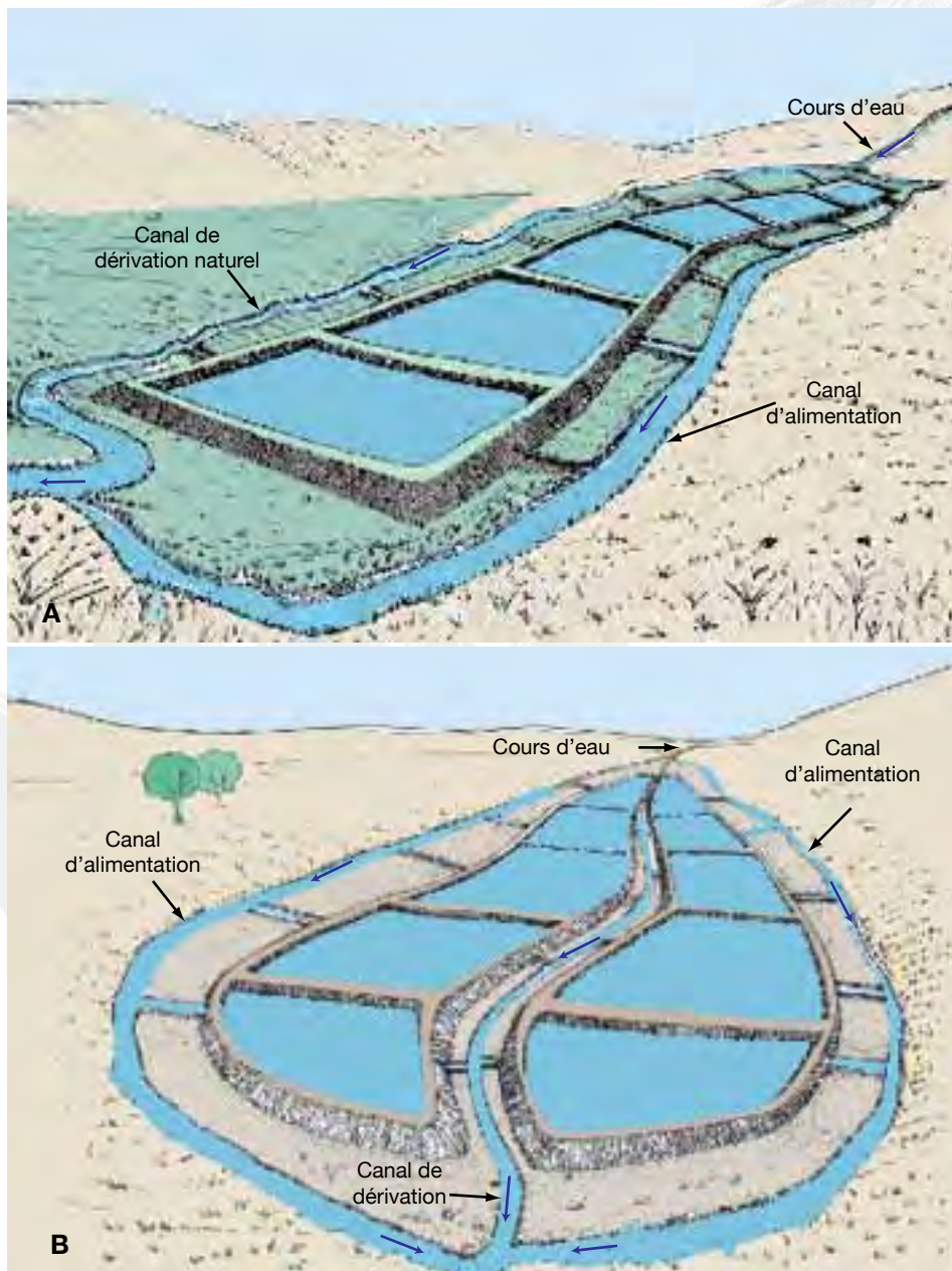
Figure 46. Exemples de système piscicole en dérivation.
