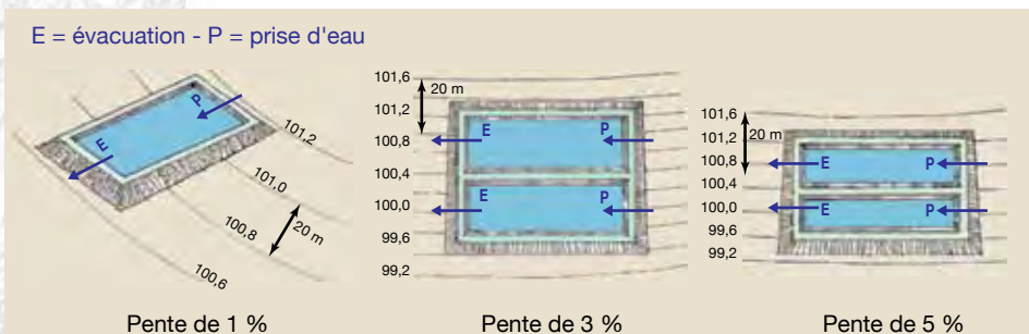
Figure 40. Disposition et forme des étangs selon la pente.
