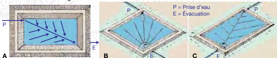
Figure 72. L'assiette. Direction de la pente (A) et disposition des drains : Rayonnant (B) ; En « arêtes de poisson » (C).
