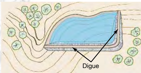
Figure 39. Exemple d'étang dont la forme est adaptée à la topographie. Ici, deux digues seulement sont nécessaires.
