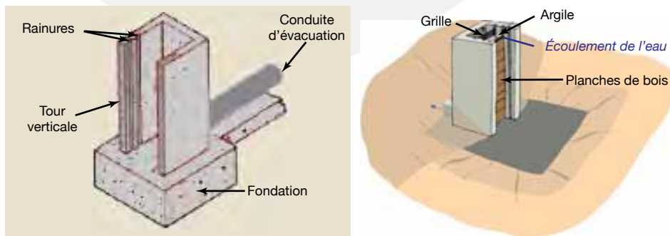
Figure 83. Composition d'un moine.
