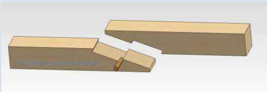
Assemblage en trait de Jupiter
