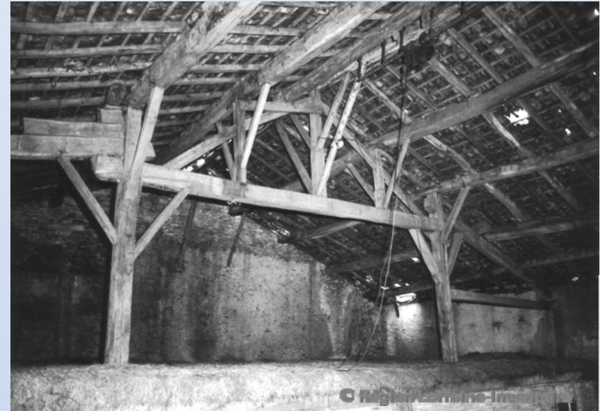
Ferme prolongée par des arbalétriers, 54-Labry.
