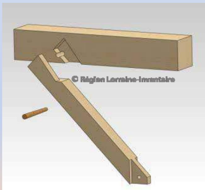
Demi-queue d'aronde à mi-bois...
