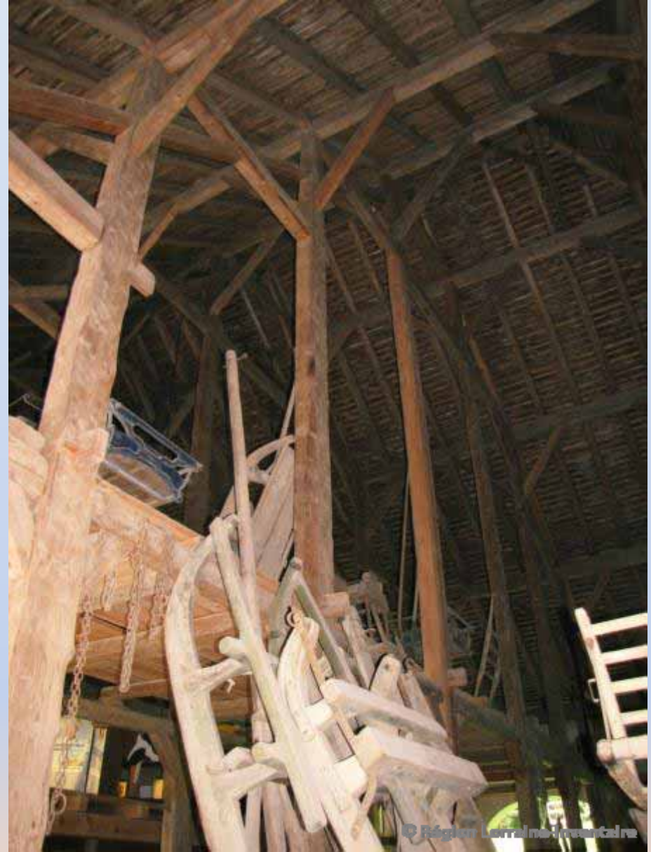
Charpente de ferme genevoise, 18 e siècle, Suisse, éco-musée de Ballemberg .
