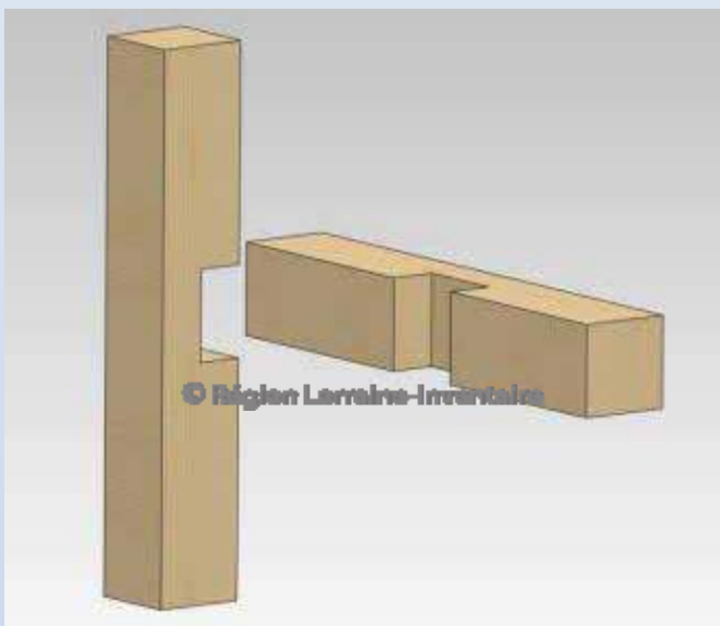
Assemblage à mi-bois
