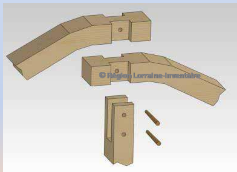
Enfourchement
