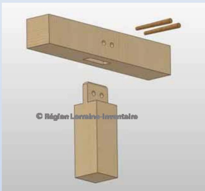
Assemblage tenon-mortaise...
