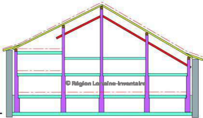
poteaux porteur de pannes
