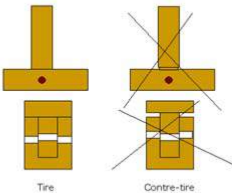
Liaisons bois sur bois
