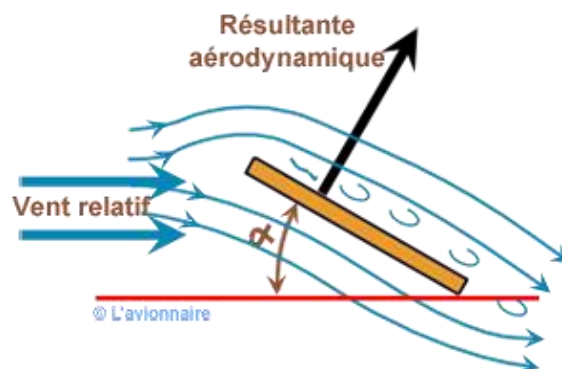
Figure 4.1. Angle d'attaque ou incidence pour une plaque plane.
