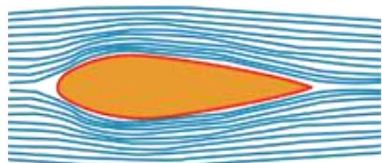
Figure 5.10 Résistance 5 %
