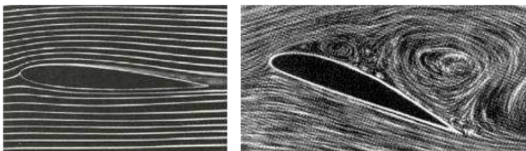
Figure 4.4. Décolage de la couche limite
