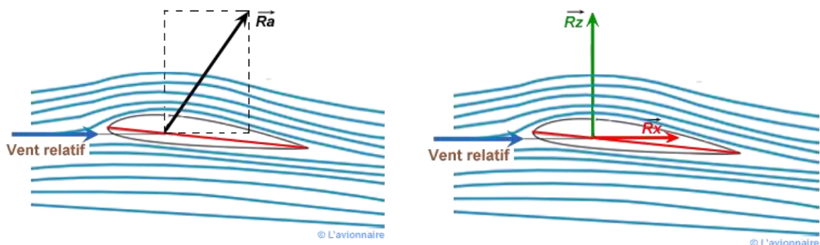
Figure 4.2. Résultante aérodynamique
